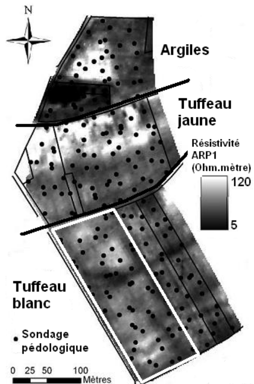
Fig. 1 : Carte de résistivité du sol, et localisation des types de substrat et des sondages pédologiques.
