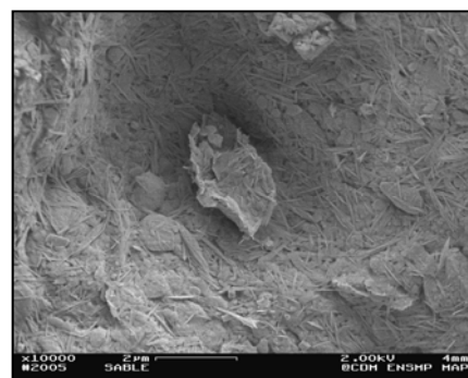
Fig. 4 : Revêtements argileux d'un grain de quartz
