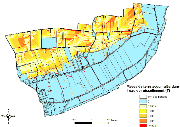
Figure 1 : Transport de matière solide au sein de la zone d'étude de Seully lors d'un événement pluvieux, août 2007
