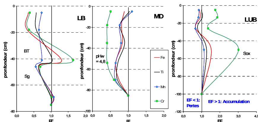
Figure 1 : Profil de FE obtenus pour Fe, Ti, Mn et Cr pour les trois pédons analysés sur diorites.
