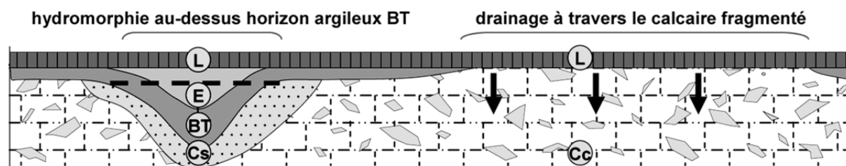
Figure 3 – Schéma du comportement différentié des structures polygonales et leurs zones périphériques à structures argileuses invaginées.
