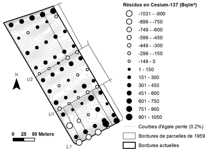
Figure 1 : Résidus* en ^{137}\text{Cs} mesurés sur l'ensemble du site d'étude et surimposés aux courbes d'égale pente.
