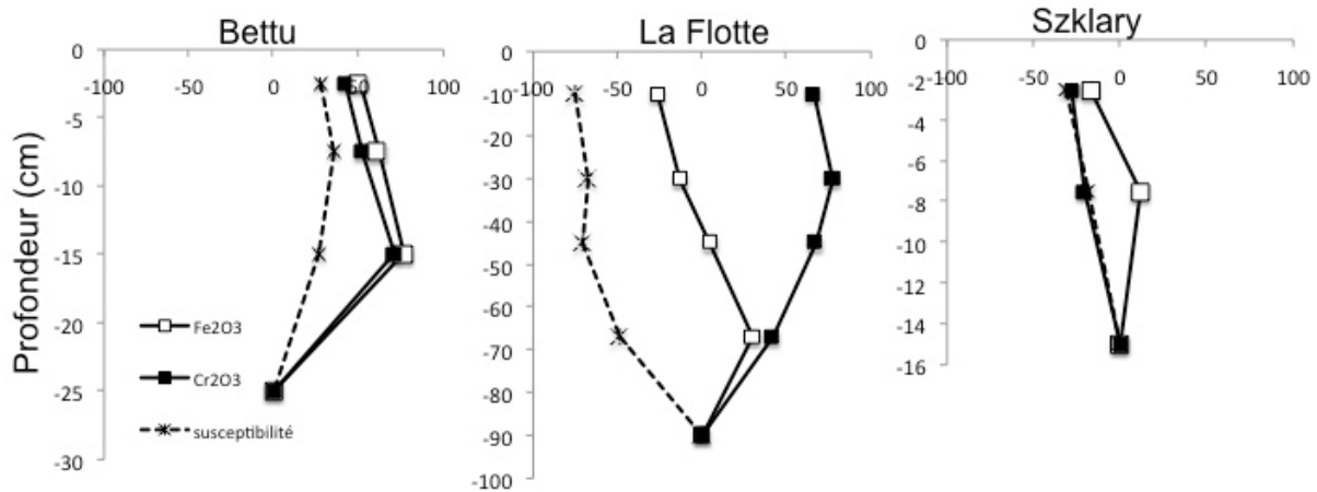
Figure 1 : Susceptibilité magnétique et bilans géochimiques des profils exprimés en %.
