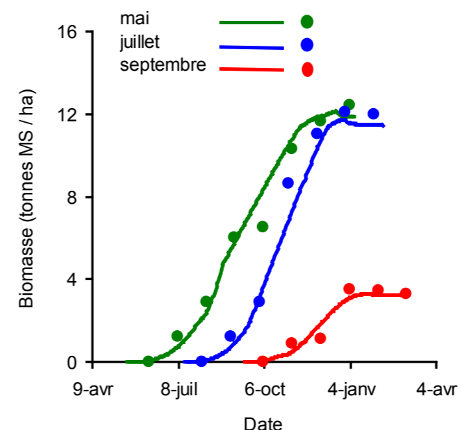
Figure 1 : Croissance de l'igname alata (variété Belep) pour trois dates de plantation en Guadeloupe. Les lignes représentent les résultats obtenus avec le modèle CropSyst-Igname et les cercles représentent les mesures réalisées.
