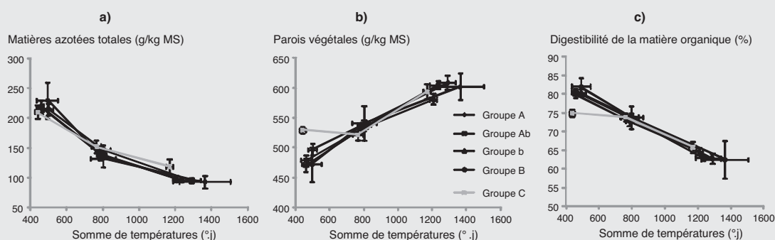
FIGURE 3 : Evolution, avec les sommes de températures au printemps, de la teneur en matières azotées totales (a), de la teneur en parois végétales (b) et de la digestibilité de la matière organique (c), pour les 5 groupes de prairies.
