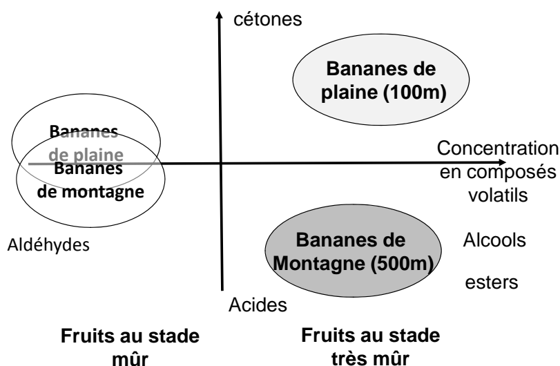
Figure 2 : Analyse en composantes principales des composés volatils de la banane
