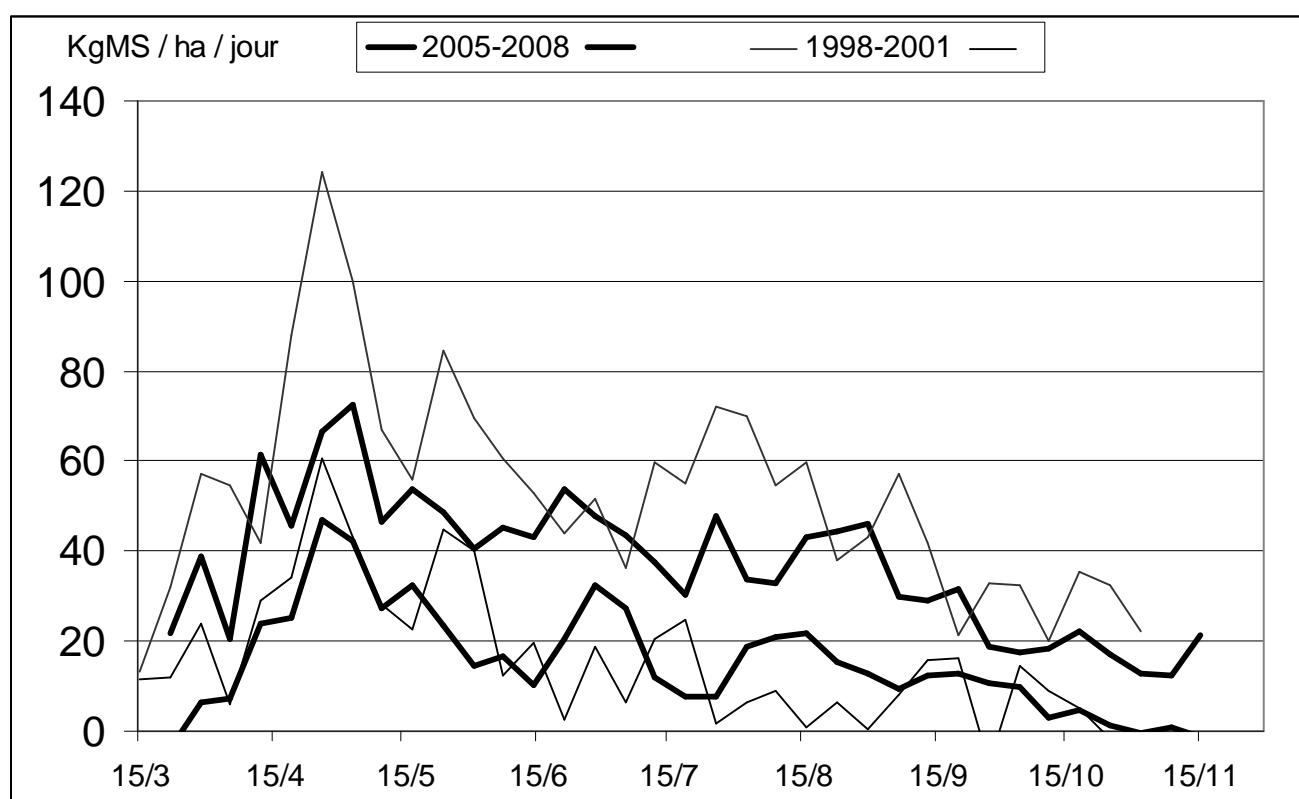
FIGURE 1 – Vitesses de croissance hebdomadaires moyennes des prairies pâturées par les vaches laitières pour les deux séries de quatre campagnes observées à Mirecourt (moyenne +/- écart-type).
