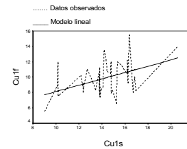
Gráfico 1.3: Variación de la Concentración de Cu en hojas frente a la concentración en suelos (ppm) en primera toma
