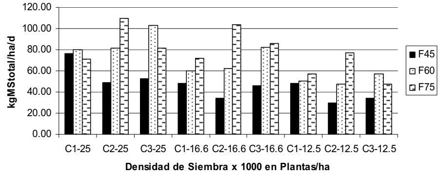
Figura 1. Comparación de las Medias de Producción Total de la Morera (kgMStotal/ha.d) en el corte 1 (C1), corte 2 (C2) y corte 3 (C3) influenciada por las densidades de siembra y frecuencias de corte.
