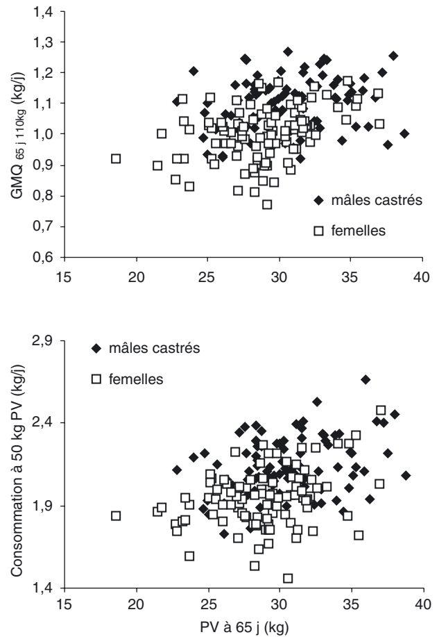
Figure 3 - Relation entre le GMQ_{65j-110kg} , la consommation à 50 kg PV et le poids vif à 65 j ( n = 192 )
