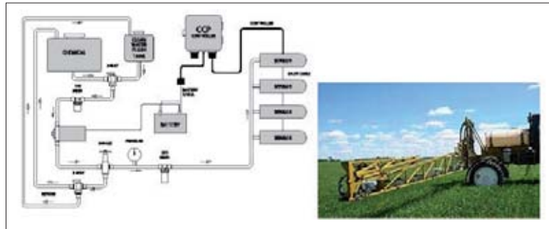
Figure 13 : Système multi capteurs « Ntechindustries » ( weedseeker)
