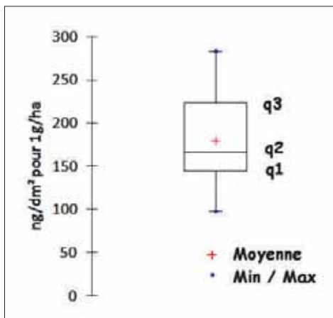
Graphique 8 : Distribution de la variable « quantité moyenne de marqueur reçue sur la vigne artificielle » (exprimée en ng/dm 2 pour 1 g/ha) pour un panel de 45 pulvérisateurs testés Distribution of the average quantity of tracer measured on the artificial vine from 45 sprayers tested
