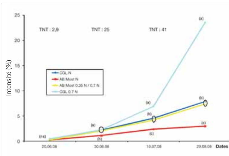
Graphique 10 : Intensité de destruction du feuillage par le mildiou en fonction du matériel et de la dose utilisés Severity of attack of downy mildew on foliage according to the sprayer and the doses used
