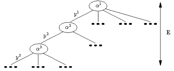
FIG. 1 – Représentation d'une politique d'échantillonnage par un arbre.
