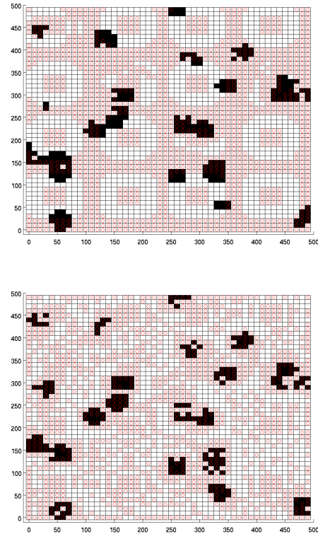
FIG. 5 – Exploration de la zone d'étude pour les échantillonnages statique (haut) et adaptatif (bas). Une croix rouge indique les sites qui ont été visités, un fond blanc indique un site pour lequel le phénomène a été reconstruit comme absent, un fond noir indique un site pour lequel le phénomène a été reconstruit comme présent ou un site où le phénomène a été observé.
