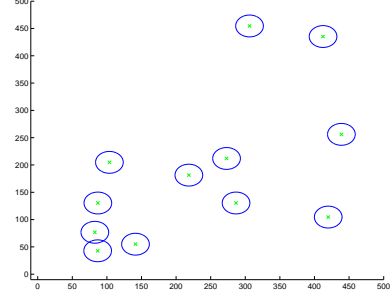
FIG. 2 – Réalisation d'un modèle booléen avec pour grain primaire un disque de rayon constant.
