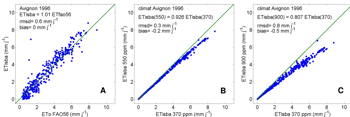
Figure 1. Comparaison des simulations de ETo en condition actuelle ([CO 2 ] a = 370 ppm) avec ISBA-A-gs par rapport à (A) EToFAO56, (B) ET simulée avec ISBA-A-gs pour [CO 2 ] a = 550 ppm et (C) 900 ppm.
