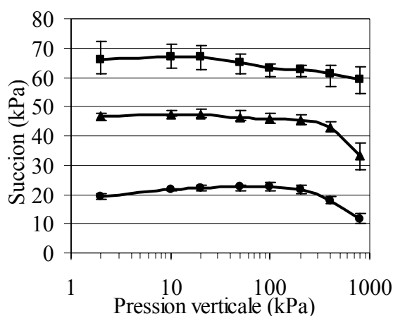
Figure 2: La variation de la succion au cours de la compression pour différentes teneurs en eau initiales: 0,198 \text{ g g}^{-1} (cercles), 0,16 \text{ g g}^{-1} (triangles), 0,143 \text{ g g}^{-1} (carrés). Les barres sont les erreurs entre trois différentes répétitions.
