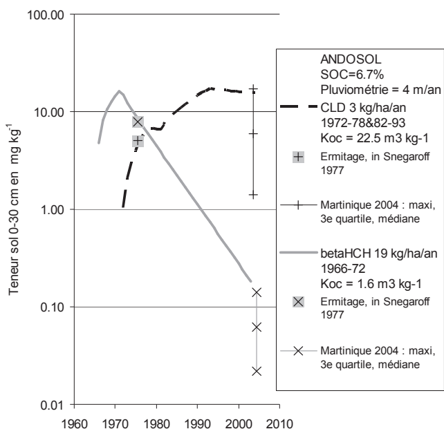
Figure 3 : Illustration des devenir en parallèle de la chlordécone et du β-HCH par le modèle WISORCH, calé sur les données de 1975 [8], validé par les bornes supérieures des analyses de 2004 en Martinique.
