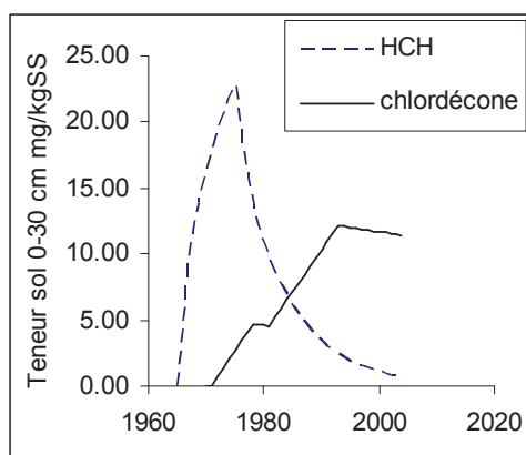
Figure 1 : Contaminations calculées par WISORCH dans un andosol sous bananeraie pérenne, après apport de 3kg/ha/an de chlordécone (1971-1978 et 1982-1993) et après apport de 12 kg/ha/an de HCH (1965-1975).
