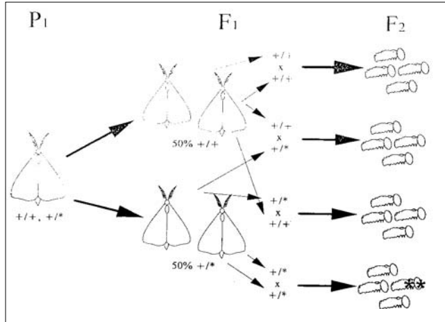
Figure 1. F 2 screen for a rare resistance allele (*). Chaque lignée isofemelle est mise en place à partir d'une femelle fécondée par un mâle, capturés directement en population naturelle ( P 1 ). Si l'un des deux parents est hétérozygote pour l'allèle de résistance (i.e. de génotype +/* ), la fréquence des larves */* lors de la deuxième génération sera de 1/16. D'après Andow & Alstad (1998).
