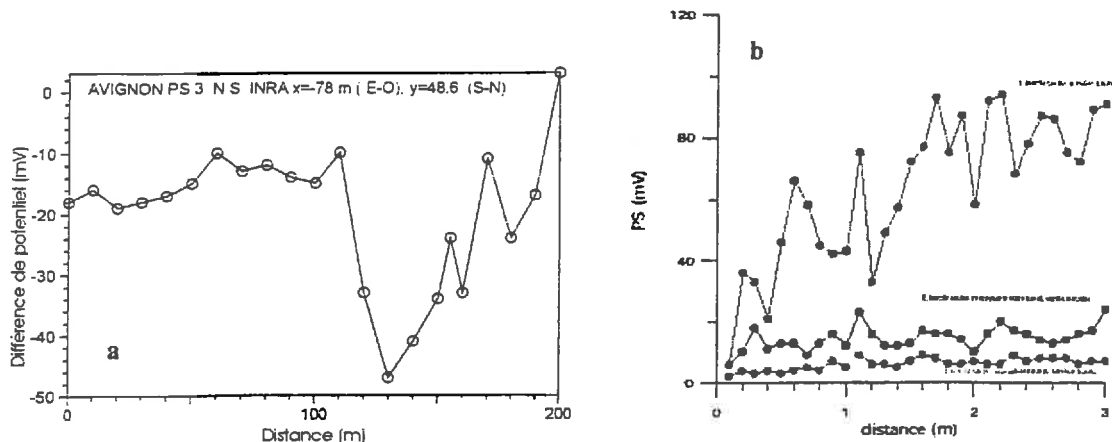
Figure 6 : Evolution de la PS mesurée en surface le long d'un transect Nord – Sud de la parcelle expérimentale en Novembre 99 (a) et Evolution de la PS sur un transect métrique en fonction de la profondeur d'enfoncement des électrodes en mars 2000 (b).
