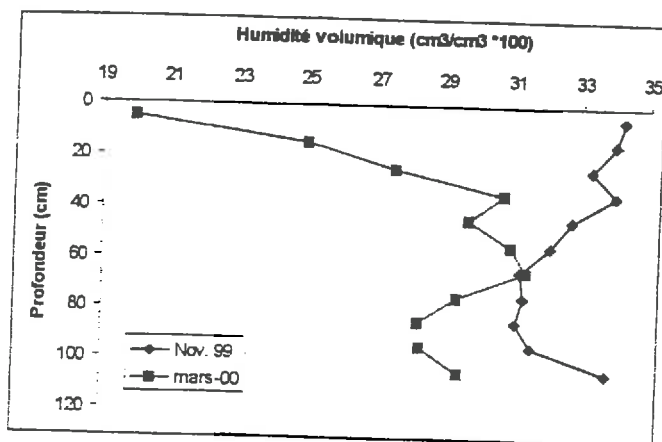
Figure 3 : Humidité volumique du sol en Novembre 99 et Mars 2000. Profils effectués à proximité du transect électrique 3D.
