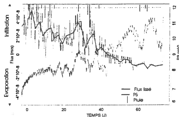
Figure 7 : Evolution du flux hydrique en non-saturé à 35 cm de profondeur dans le cas d'un sol limoneux et variations de PS mesurées entre 30 et 40 cm de profondeur ( Temps 0 = 1 janvier 2000).
