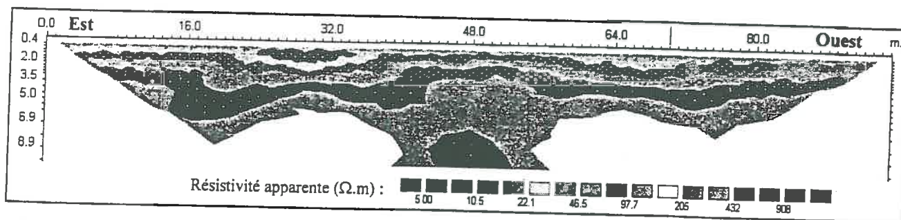
Figure 4 : Exemple de données de résistivité apparente d'un transect électrique 2D multinode (Est-Ouest ici)
