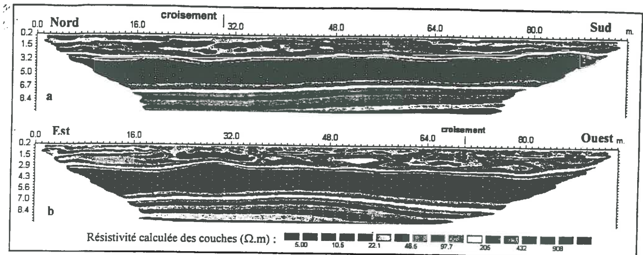
Figure 5 : Résistivité calculée par inversion des couches de sol d'un transect électrique Nord-Sud (a) et Est-Ouest (b).
