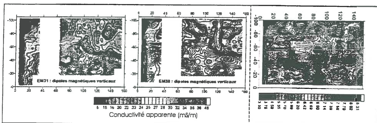
Figure 1 : Cartographie de la conductivité apparente EM38 et EM31 du site expérimental en novembre 99 et mars 2000.
