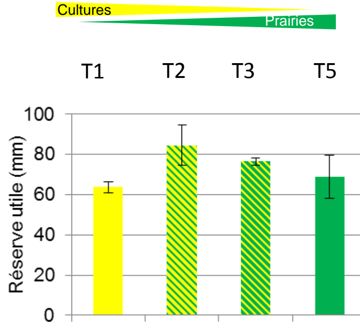
Evolution du Réservoir Utilisable dans les deux premiers horizons du sol
