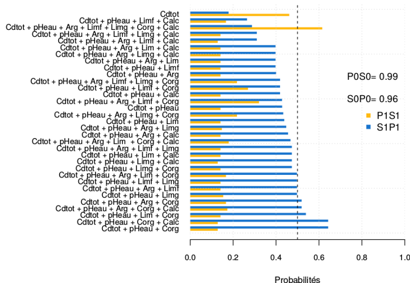
Figure 1 : Performances de différents modèles logistiques à prédire la probabilité de non conformité d'un échantillon de blé dur (=teneur en Cd dépassant le seuil réglementaire de 0,2 mg Cd/kg).
