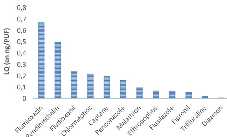
Figure 2 : Limites de quantification (LQ) obtenues par GC-MS/MS
