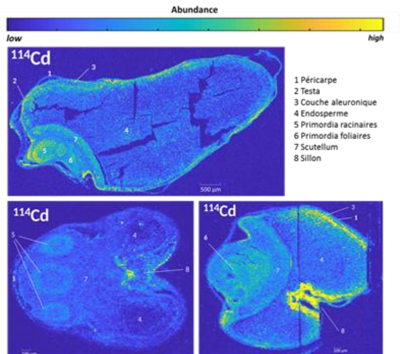
Figure 2. Cartes de localisation de Cd dans un grain de blé dur (cv. Sculptur ) obtenues par LA-ICP-MS à partir d'une coupe longitudinale et de deux coupes transversales. A noter que les 3 plans de coupe traversent l'embryon. Les grains utilisés ont une teneur totale en Cd avoisinant les 1.5 µg Cd g -1 .
