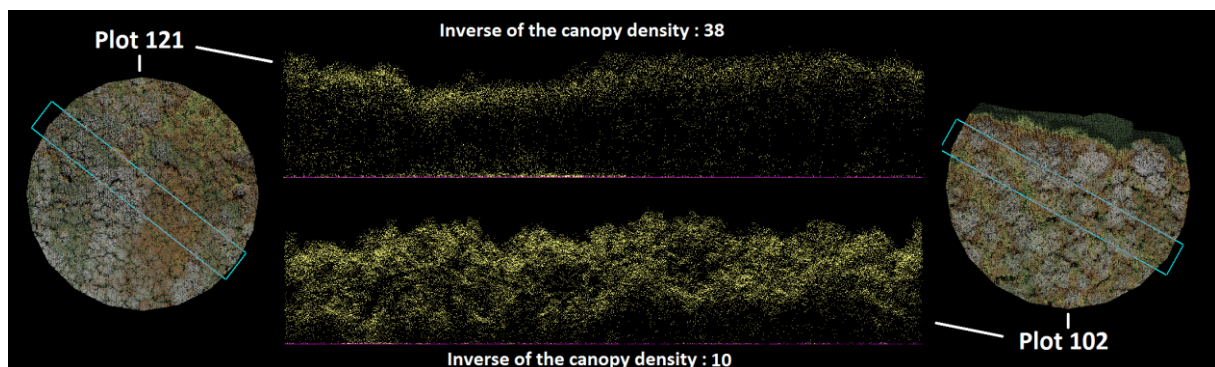
Figure 36 Visualisation des données LiDAR pour deux plots présentant des valeurs extrêmes de la couverture de canopée.
