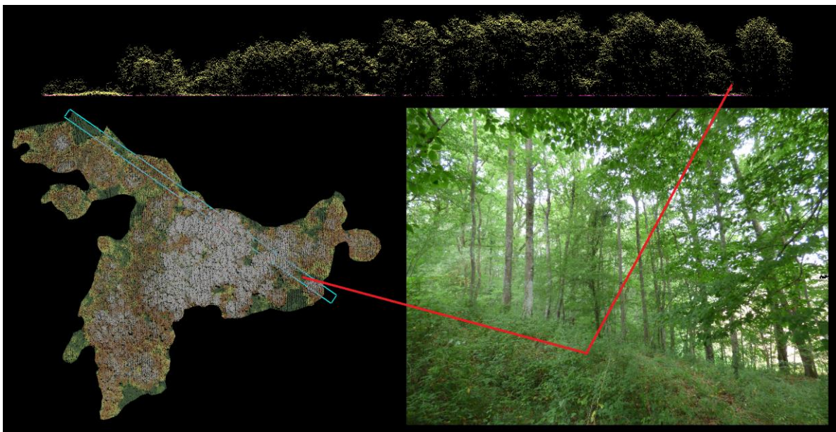
Figure 24 Photographie terrain et coupe verticale du nuage de points.
