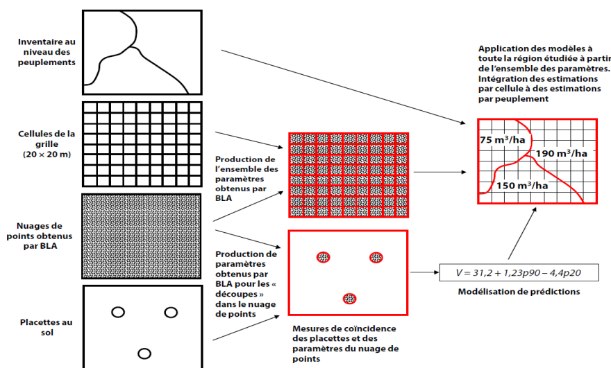
Figure 5 Schéma de l'approche par zone tiré de White et al. (2013) : calibration de modèles prédictifs à partir des relevés terrains des placettes et construction d'une grille dans laquelle les variables LiDAR obtenues par balayage laser aéroporté (BLA) vont être extraites pour chaque cellule de la taille des placettes afin de prédire la variable dendrométrique d'intérêt sur toute la zone d'étude.
