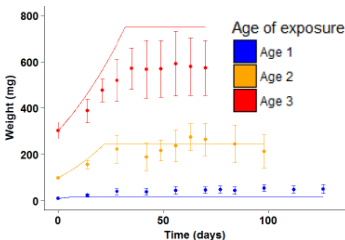
Figure 4 : Courbes de croissance d'individus juvéniles d' A. caliginosa de trois âges différents exposés dans un sol contaminé à 77.5 \text{ mg kg}^{-1} de cuivre. Les lignes représentent le modèle et les points sont les données.
