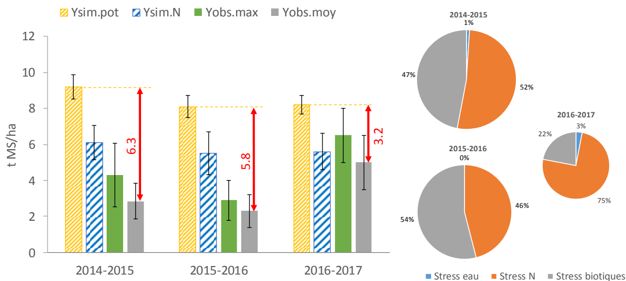
Figure 1 : Rendements potentiels simulés par STICS, rendements réels moyens et maximaux observés, et yield gap pour le blé (en rouge). Valeurs moyennes et écart-type entre parcelles.
