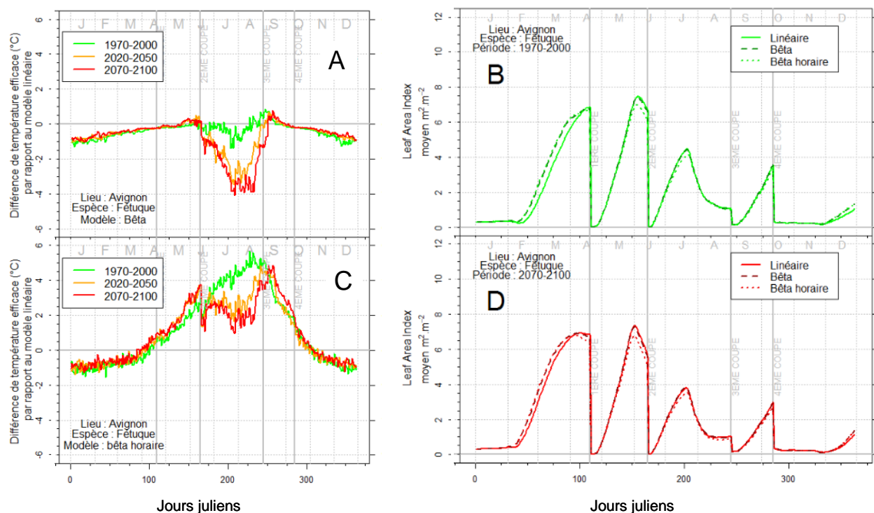
Figure 1 : Modifications des températures efficaces (moyennes sur 30 ans) liées au changement du formalisme de réponse à la température pour la fétuque à Avignon (A et C) et impacts sur la dynamique du LAI (B et D).
