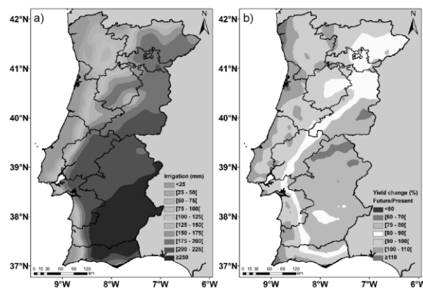
Figure 2 : (a) Quantité d'eau d'irrigation (mm) nécessaire à l'avenir (2040-2070) pour maintenir les rendements actuelles. (b) Proportion (%) d'évolution du rendement entre le futur (avec irrigation, 2040-2070) et le présent (sans irrigation, 1980-2005).
