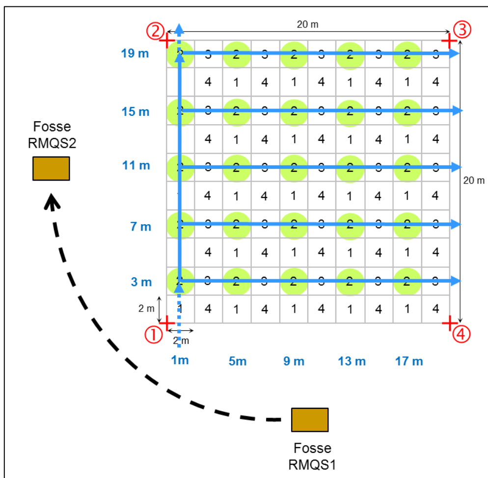
Figure 6 – Principe de jalonnement des points de prélèvement de la surface d'échantillonnage à partir du câble et implantation de la fosse RMQS2
