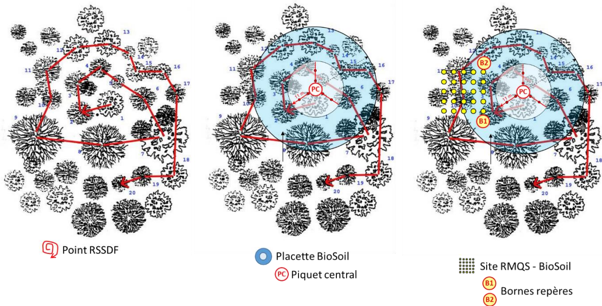
Figure 10 – Point du réseau systématique de suivi des dommages forestiers (RSSDF), placette BioSoil et site RMQS-BioSoil, avec leurs points de repère respectifs
