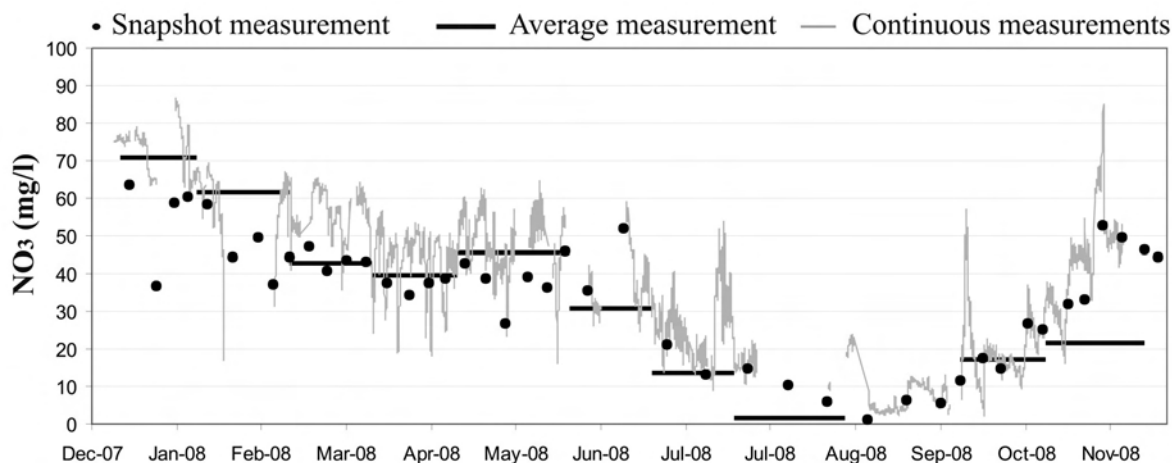
Figure 4.2. Comparaison de trois types de mesures des concentrations de NO 3 - , ponctuel, moyenné (SC Sampler) et continu. Source : Rozemeijer et al. , 2010. © American Chemical Society
