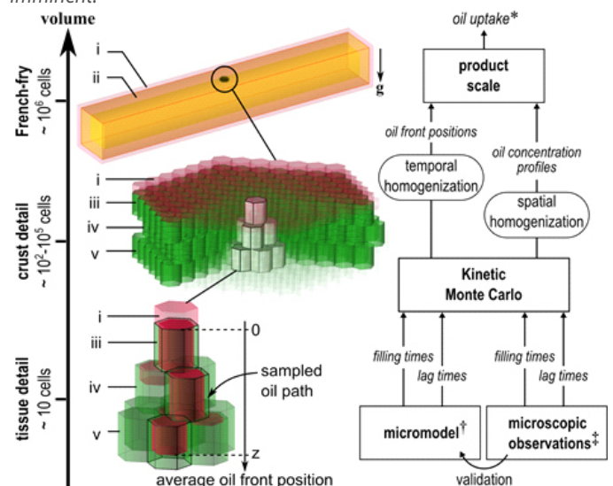
Principes de la modélisation et simulation multiéchelles de la prise d'huile dans une frite réelle. Principles of multiscale modeling and simulation of oil uptake in a real French-fry.
