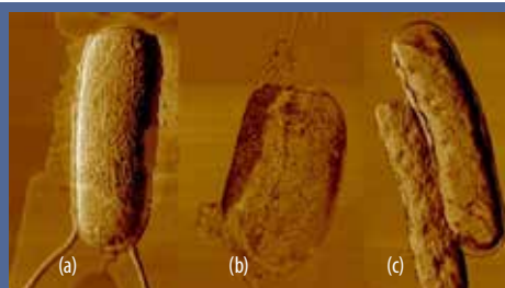
Effets du lysozyme sur les membranes d' E. coli visualisés par microscopie à force atomique / Effects of lysozyme on E. coli membranes by AFM (a) E. coli K12, (b) with native lysozyme, (c) with dry-heated lysozyme
