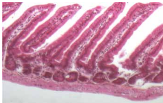
Expression protéines intestinales dans le petit intestin de souris / Intestinal proteins expression in mouse intestine © Inra
