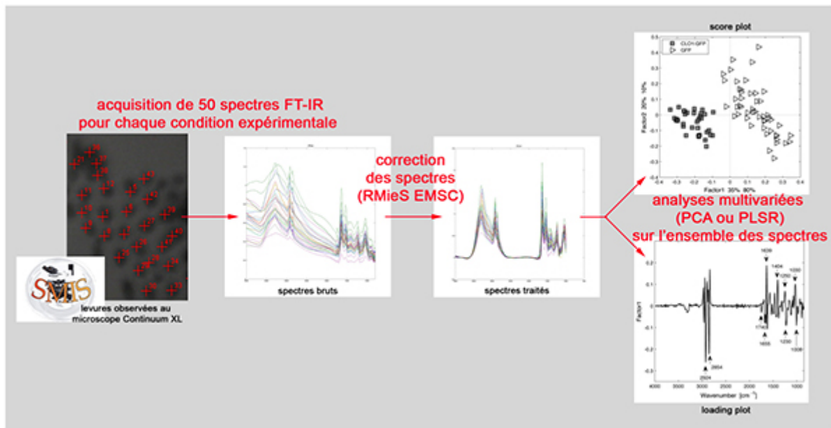
Figure 2 : chaîne d'acquisition et de traitement des données
