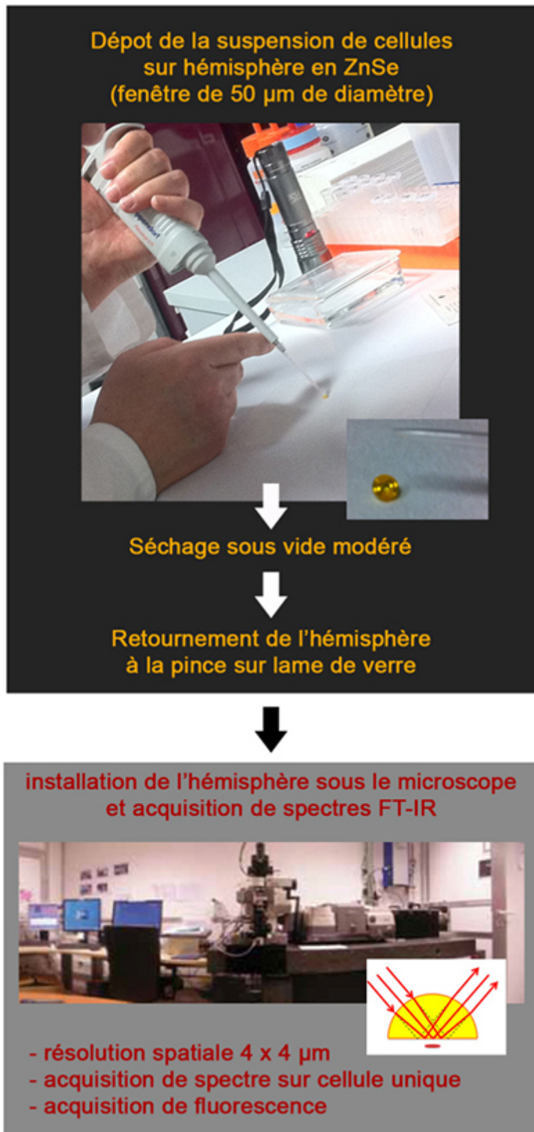
Figure 1 : prise de vues de la ligne et du dépôt sur hémisphère
