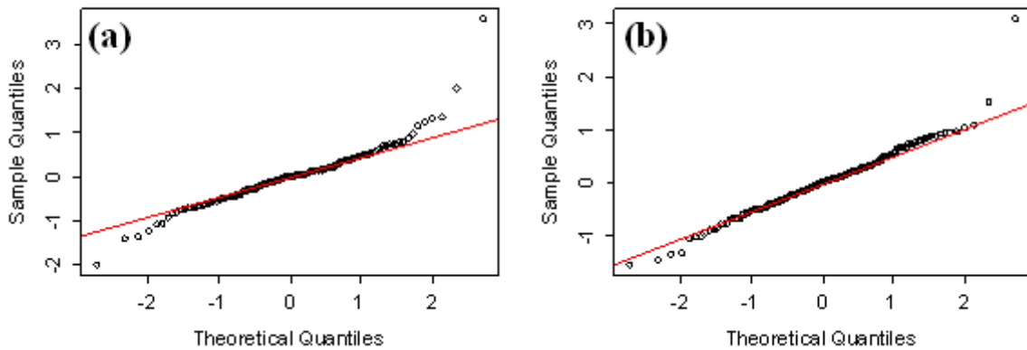
Figure 16 : Q-Q plot des résidus pour le modèle avec effet fixe occupation sans (a) et avec (b) transformation de Box-Cox du nickel pour la couche de surface
