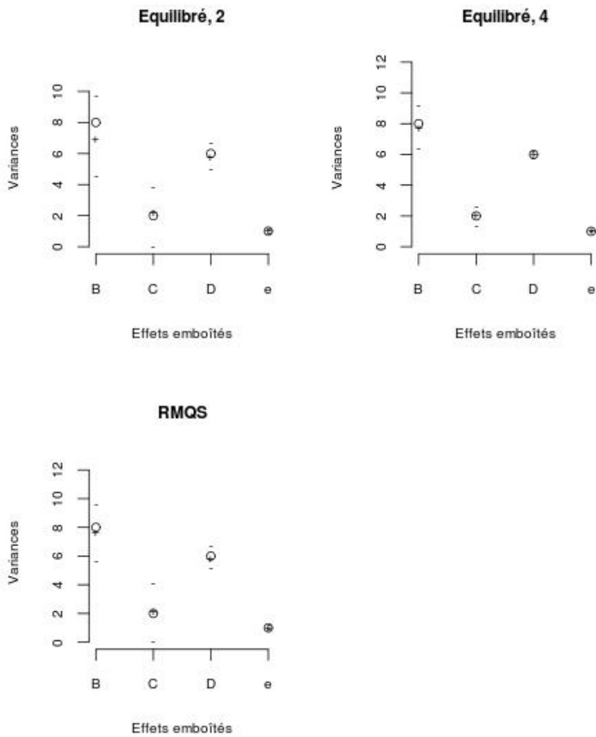
Figure 5 : Comparaison des moyennes des variances estimées pour 1000 réplicas avec la variance imposée v_2 = (5, 8, 2, 6,1) . Variance imposée et moyenne de la variance estimée par simulation pour chaque composante représentée respectivement par un cercle et une croix. Le 1 er et 9 ème décile représentés par un trait.
