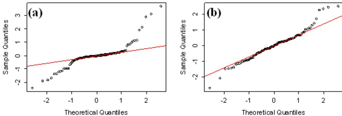
Figure 17 : Q-Q plot des résidus pour le modèle sans effet fixe, sans (a) et avec (b) transformation de Box-Cox du cobalt pour la couche de sub-surface.
