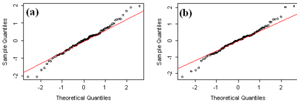
Figure 13 : Diagrammes Q-Q des résidus pour les modèles sans effet fixe (a) et effet fixe site (b) du plomb pour la couche de sub-surface.
