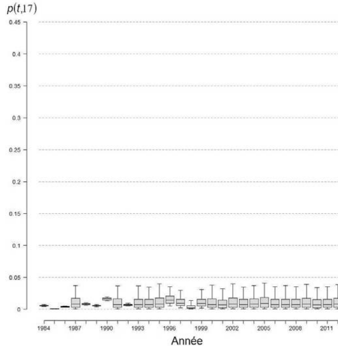
Figure A17.2. Évolution de 1984 à 2012 des probabilités de retour dans la rivière Aux Plats pour les adultes de la métapopulation de saumon atlantique ( Salmo salar L.) de l'île d'Anticosti (Québec). Boxplots : percentiles 5, 25, 50, 75 et 95 des distributions marginales a posteriori issues du modèle sur la dynamique de renouvellement de la métapopulation.
