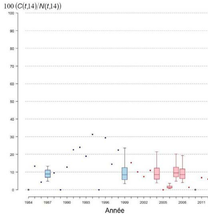
Figure A14.4. Évolution de 1984 à 2012 des taux d'exploitation par la pêche sportive dans la rivière Ferrée (île d'Anticosti, Québec). Box-plots : percentiles 5, 25, 50, 75 et 95 des distributions marginales a posteriori issues du modèle sur la dynamique de renouvellement de la métapopulation de l'île d'Anticosti ; points données ; étoiles : années pour lesquelles l'effort de pêche est égal à 0 ; couleur bleue : tous les individus sont ciblés par la pêche ; couleur rouge : seuls les individus de moins de 63 cm sont capturés, les autres étant remis à l'eau.
