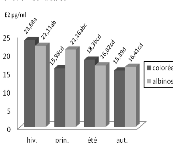
Figure 2 : Taux de E2 chez les deux phénotypes en fonction de la saison
