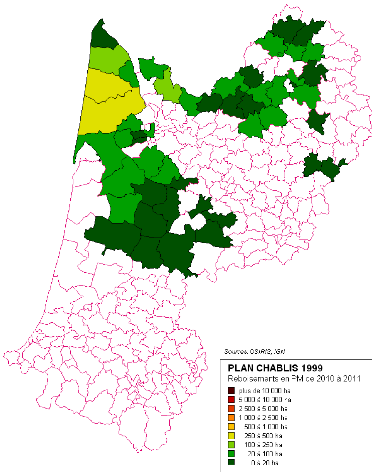
10 - Reboisements en Pin maritime subventionnés dans le cadre du Plan chablis 1999 enregistrés sous OSIRIS en 2010 et 2011
