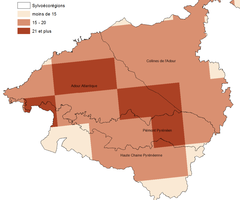
36 - Nombre de types forestiers cartographiés par maille de 400 km 2
