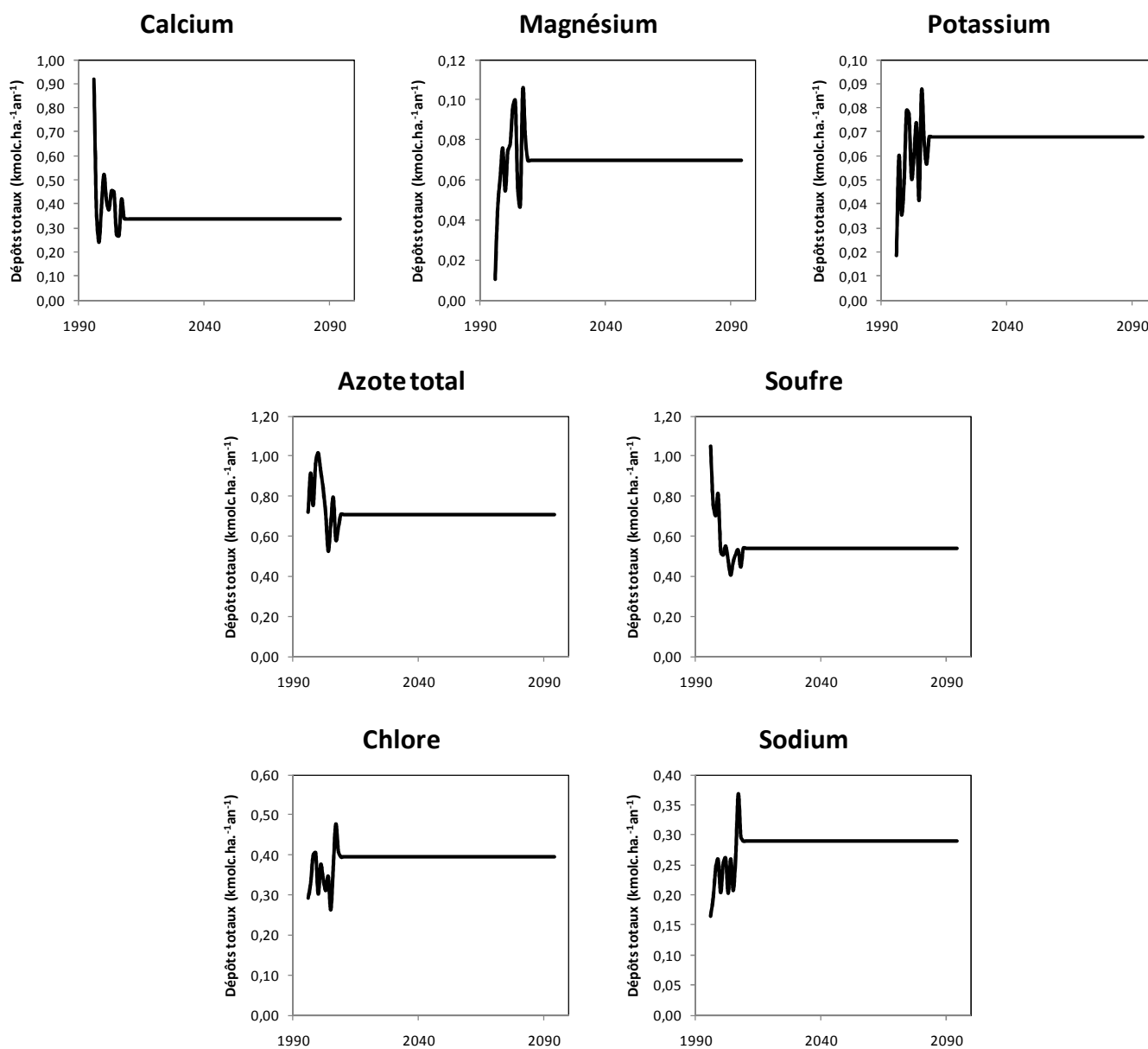
Graphique 15 : Evolution des dépôts atmosphériques totaux dans le scenario (A), niveau de dépôts constants pendant 100 ans et égal au niveau actuel, les dépôts atmosphériques totaux sont exprimés en \text{kmolc.ha}^{-1}.\text{an}^{-1}
