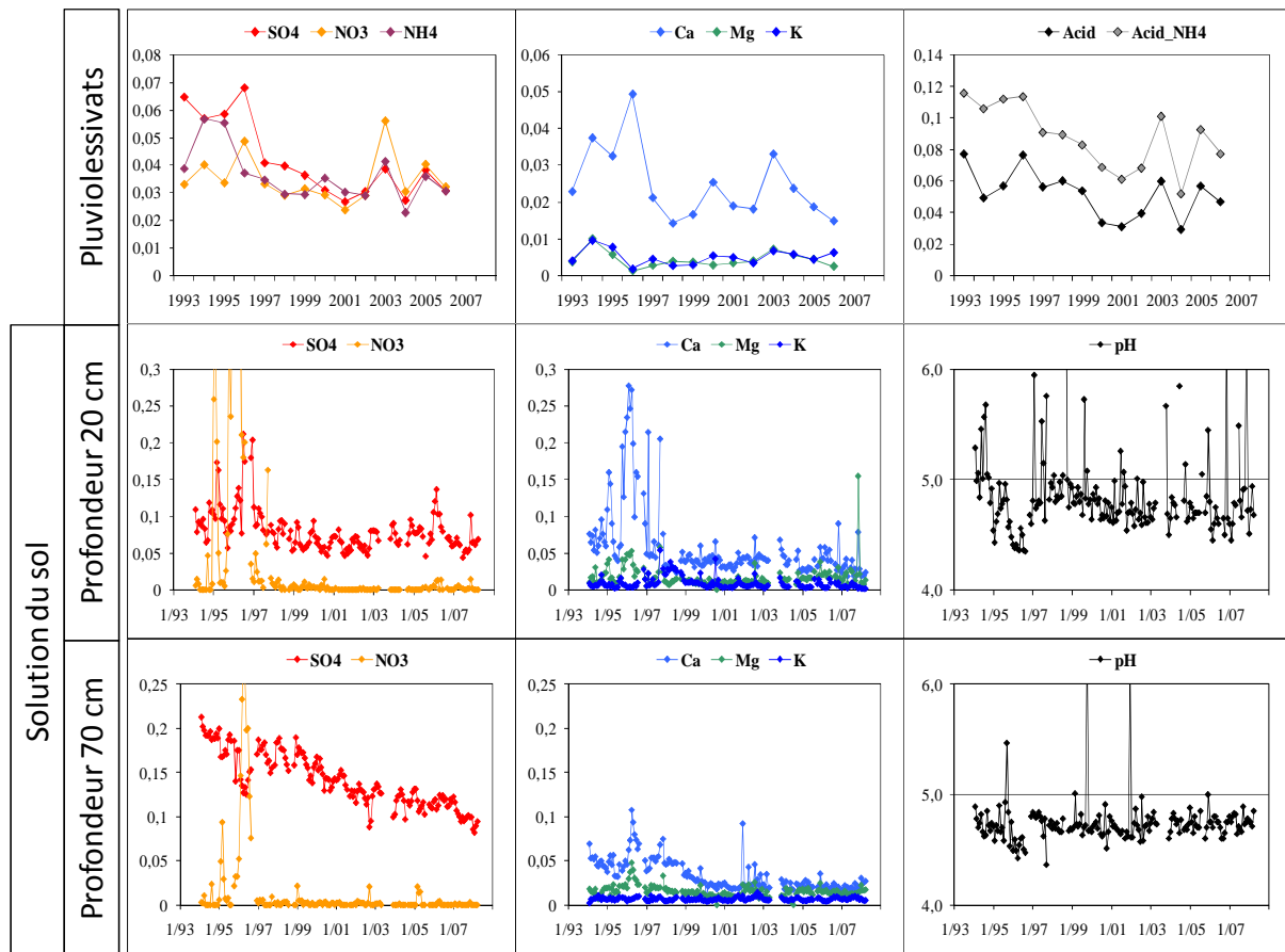
Graphique 2 : Suivi des concentrations dans les pluviollessivats et dans les solutions de sol à 20 cm et à 70 cm de profondeur pour les éléments majeurs (SO 4 , NO 3 , Ca, Mg et K). Suivi de l'acidité de ces solutions sur la période 1993-2007 pour les pluviollessivats et sur la période 1994-2007 pour les solutions du sol (bougies poreuses mises en place en décembre 1992). Les concentrations et l'acidité des dépôts sont exprimées en mmolc.l -1
