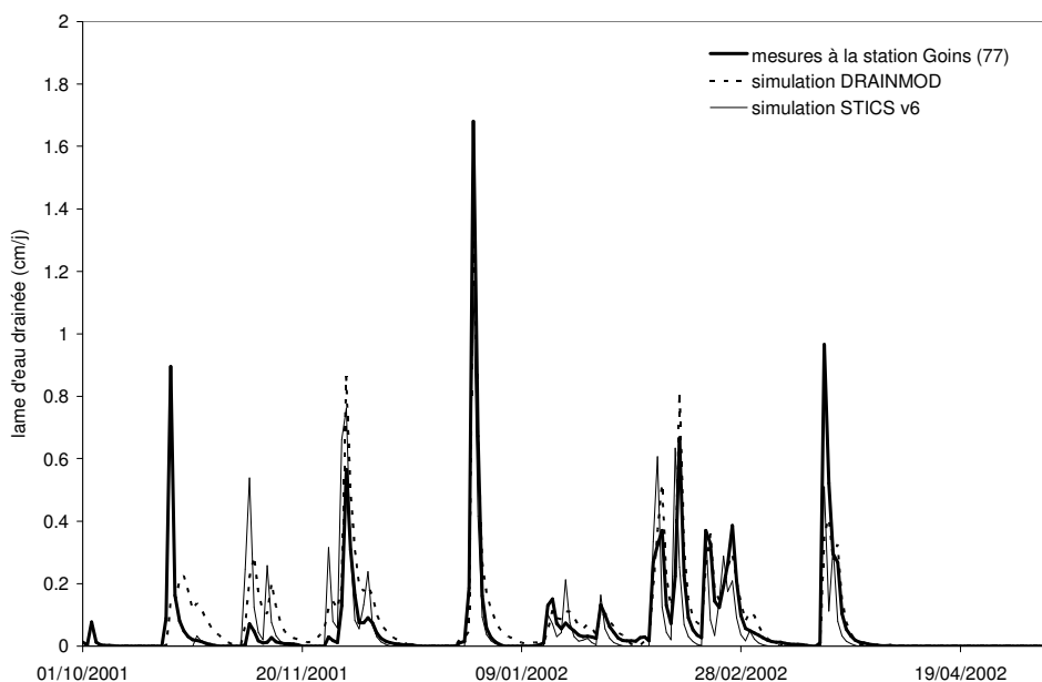
Figure 3 : Comparaison des débits mesurés à la station de Goins (Seine et Marne, 130ha) et simulés (DrainMod version 5, STICS version 6) d'octobre 2001 à mai 2002.
