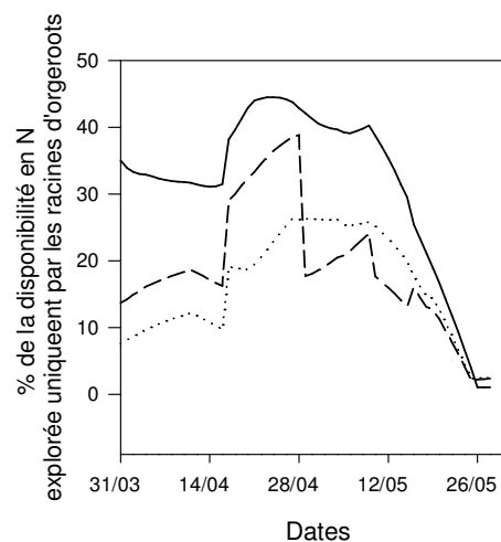
Figure 2 : Pourcentage d'azote minéral disponible pour les racines d'orge en fonction du niveau de disponibilité en azote (faible :---, moyenne :..... et forte : - - -)
