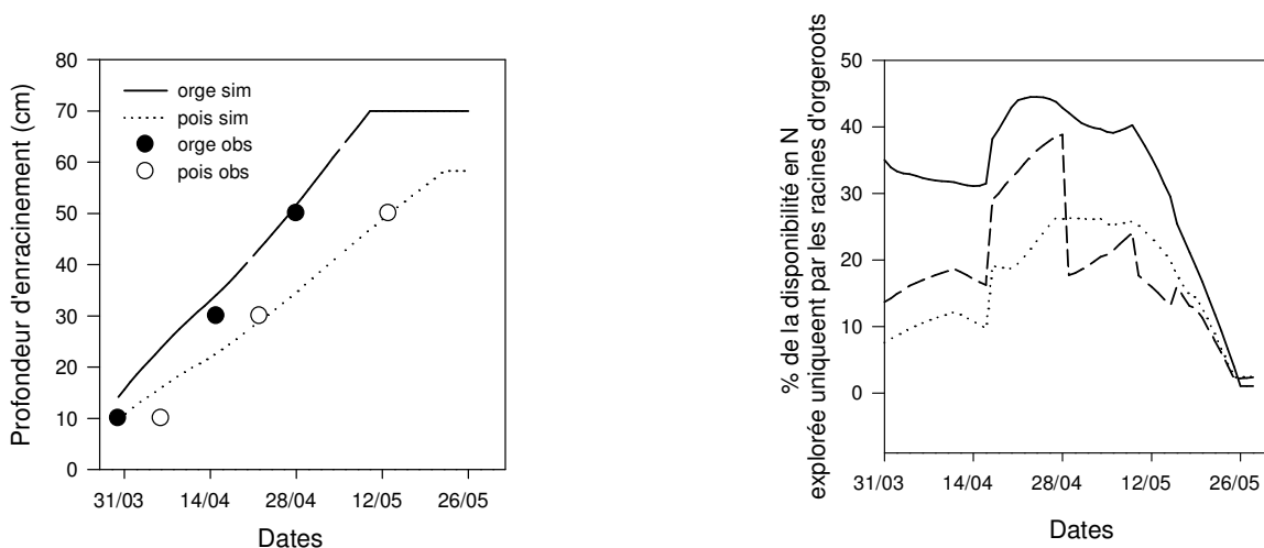
Figure 1 : Evolution de la profondeur d'enracinement du pois et de l'orge associés (observations et simulations)
