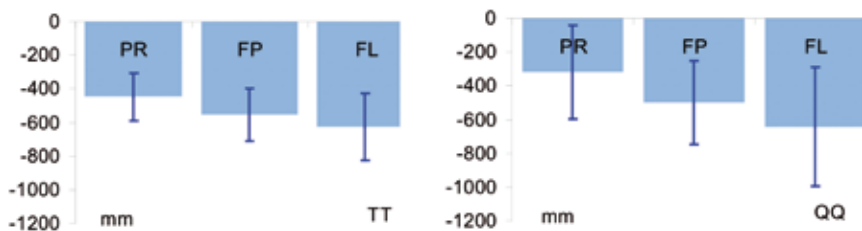
Figure 2 : déficit hydrique climatique (pluies-ET0) annuel dans le PR, le FP et le FL, à Avignon. ARPÈGE A1B*. Méthodes de régionalisation : TT (à gauche) et QQ (à droite).
