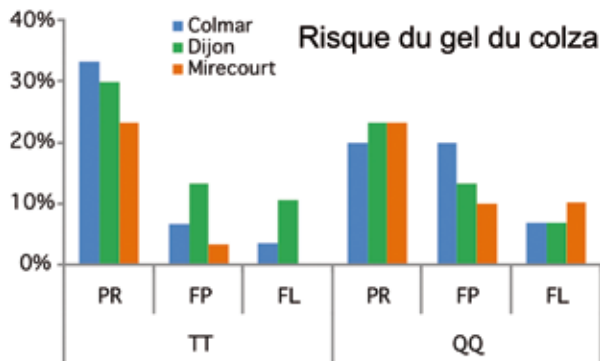
Figure 7 : évolution des risques de gel légal du colza pour deux méthodes de régionalisation du climat.
