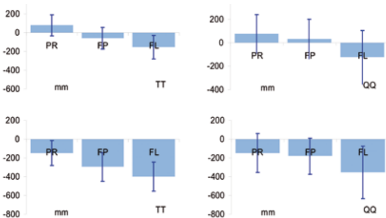
Figure 2 : déficit hydrique climatique (pluies-ET0) annuel dans le PR, le FP et le FL à Clermont-Theix (en haut) et à Saint-Étienne (en bas). ARPÈGE A1B. Méthodes de régionalisation : TT et QQ.
