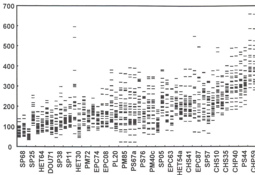
Fig. 3 : réserves utiles en eau (mm) calculées pour les deux fosses de chacune des placettes du sous-réseau météorologique forestier selon plusieurs fonctions de pédotransfert
