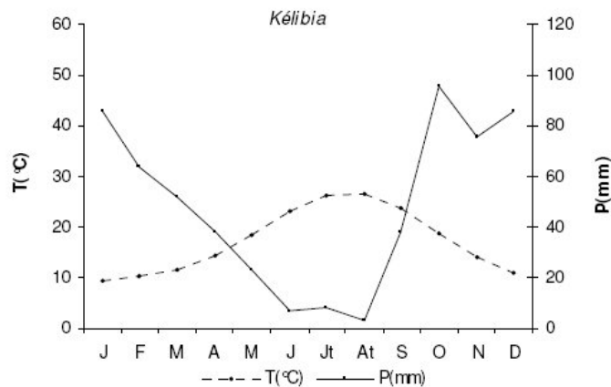
Fig.13 : Diagramme ombrothermique de Kélibia (près de Kamech, Mekki, 2003)
