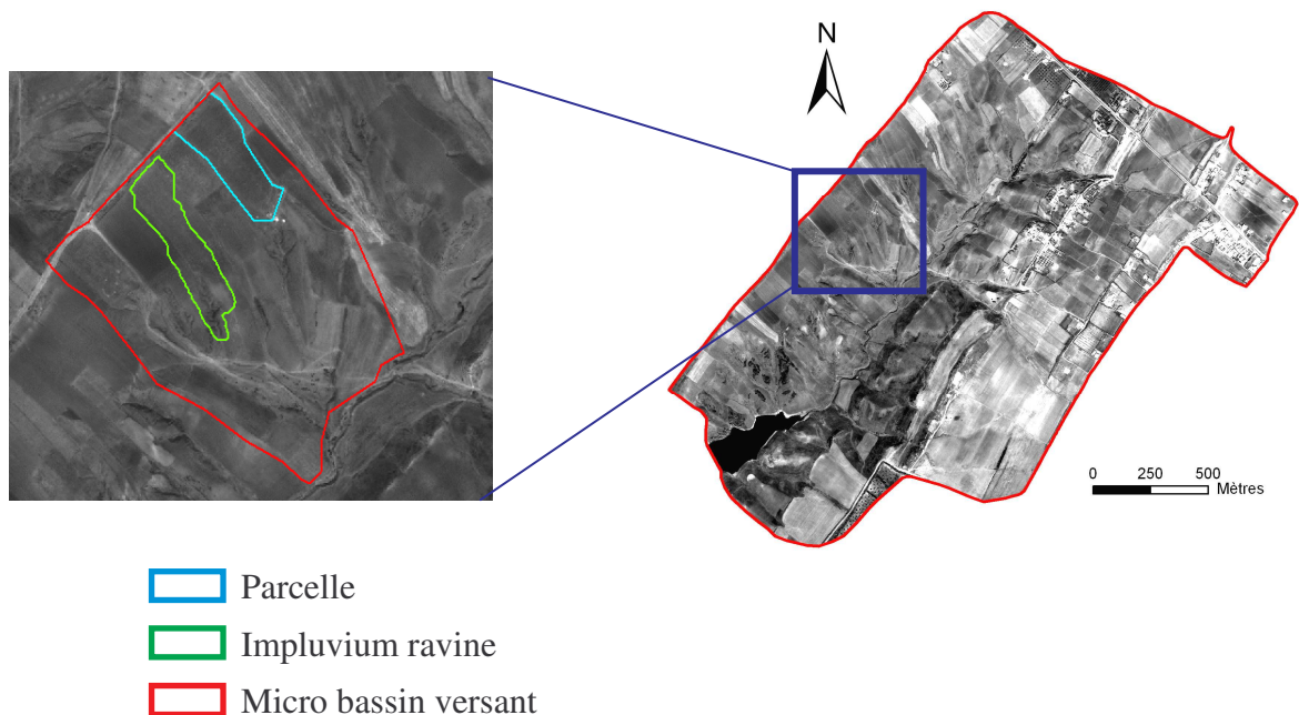
Fig.36 : Localisation des surfaces de validation
