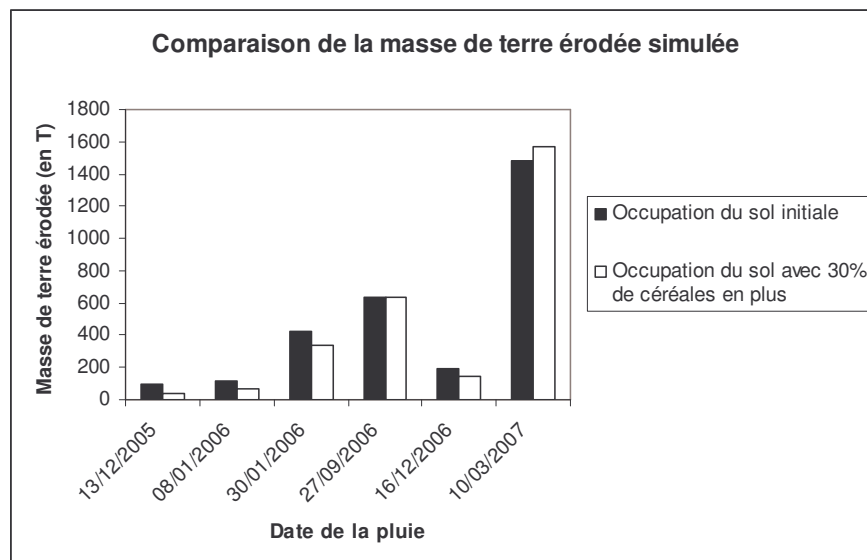
Fig.49 : Comparaison de la masse de terre érodée simulée à l'exutoire entre l'occupation initiale et l'occupation du sol avec 30% de céréales en plus
