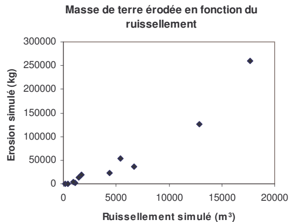
Fig.22 : Relation entre la masse de terre érodée et le volume ruisselé à l'exutoire (simulation effectuée avec la durée efficace à 5 mm/h)
