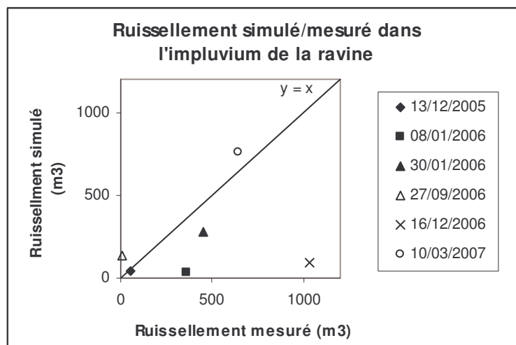
Fig.40: Résultats des simulations sur l'impluvium de la ravine
