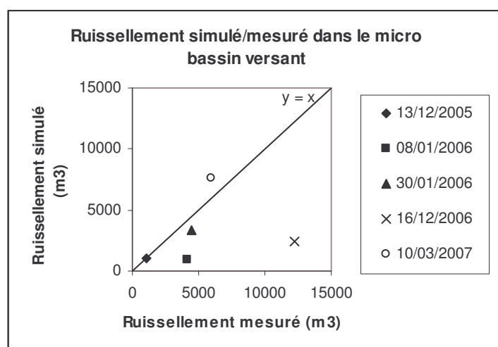
Fig.39 : Résultats des simulations sur le micro bassin versant
