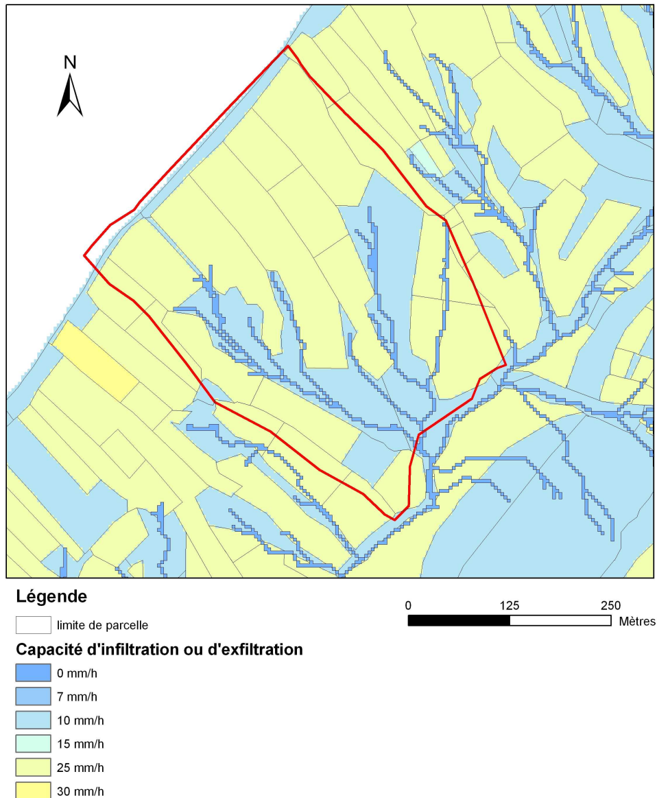
Fig.47 : Capacité d'infiltration pour la pluie du 08/01/2006 sur le micro-bassin versant.
