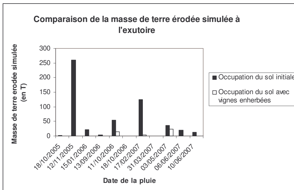
Fig.35 : Comparaison de la masse de terre érodée simulée à l'exutoire entre l'occupation du sol initiale et l'occupation du sol avec vignes enherbées
