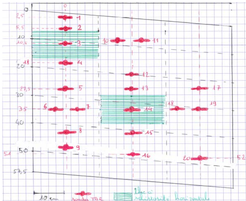
Figure 8 ; schéma d'une face latérale de la cuve, avec l'emplacement des sondes.
