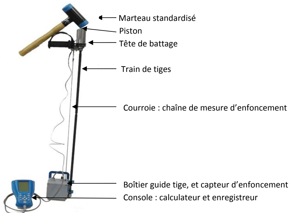
Figure 4 : photo d'un pénétromètre
