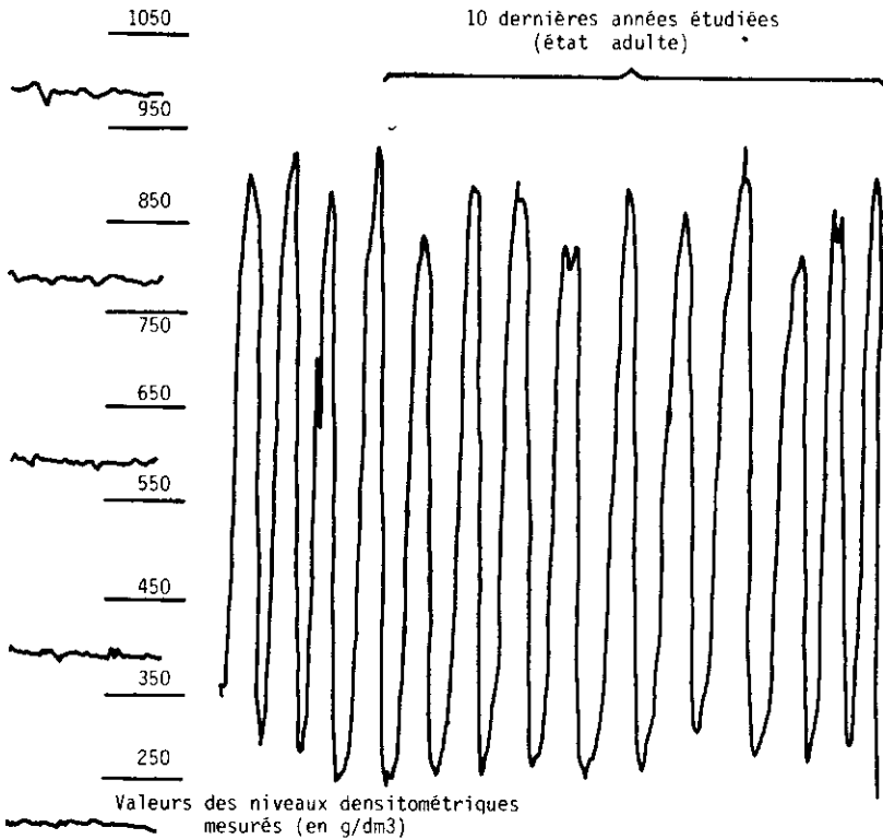
LES POLYMERES VEGETAUX Vol. 2 - part 1 Fig. 5 - Profil de densité des 10 dernières années, près de l'écorce à l'état adulte (65 ans), d'un Douglas ( Pseudotsuga Menziesii ). La figure correspond à l'état juvénile du même arbre.
