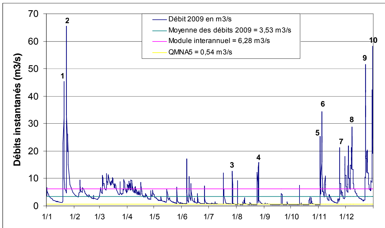
Figure 18 Positionnement des principales crues de la Leyse
