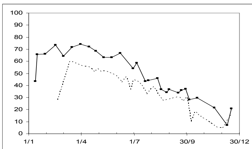
Figure 13 Variation saisonnière des concentrations en oxygène (% de la saturation) à 130 m au point B en 2009 et comparaison avec 2008 (---)
