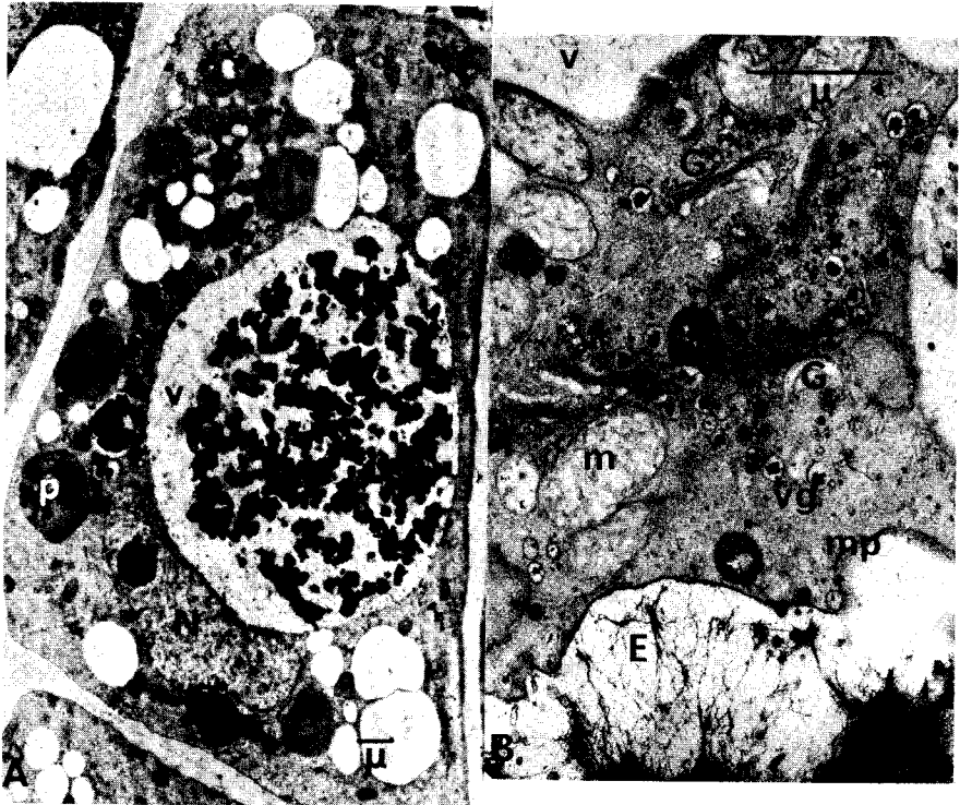
Fig. 14 — Cellules sécrétrices. A : cellule à tanins de Pommier; ceux-ci apparaissent sous forme de précipités denses dans la vacuole v. B : cellule d'Oeillet sécrétant des polysaccharides; ceux-ci, contrastés par la réaction PATAg (cf Roland, chapitre suivant), apparaissent noirs sur la micrographie. E : espace entre la paroi et la membrane plasmique mp. Autres légendes : cf. 9 et 10.
