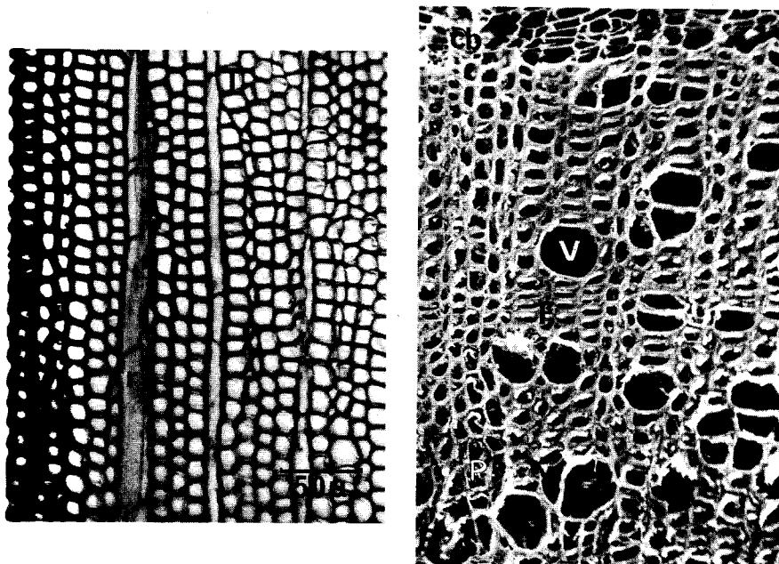
Fig. 18 — Aspect en coupe transversale de bois différents. A : bois homoxylé de Pin à crochets; r : rayon de parenchyme horizontal; T : trachéide. B : bois hétéroxylé de Sureau avec des gros vaisseaux V, des fibres F et des cellules de parenchyme P de plus faible diamètre; cb : cambium. (Cliché J.C. Roland obtenu par microscopie à balayage).
