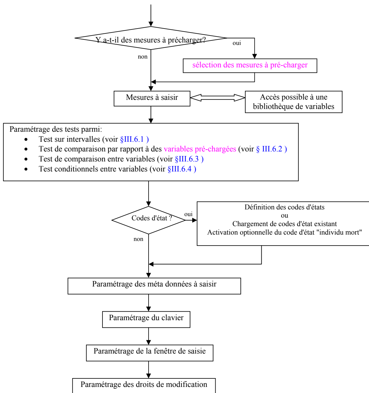
Figure 22: séquencement de la section 'variables'
