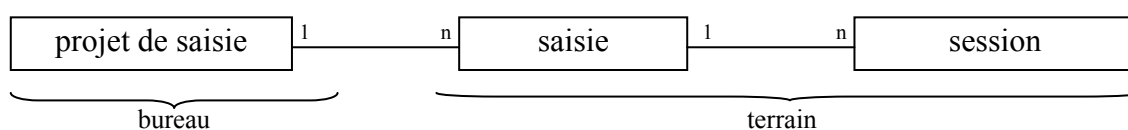
Figure 37: Liens entre projet de saisie, saisie et session
