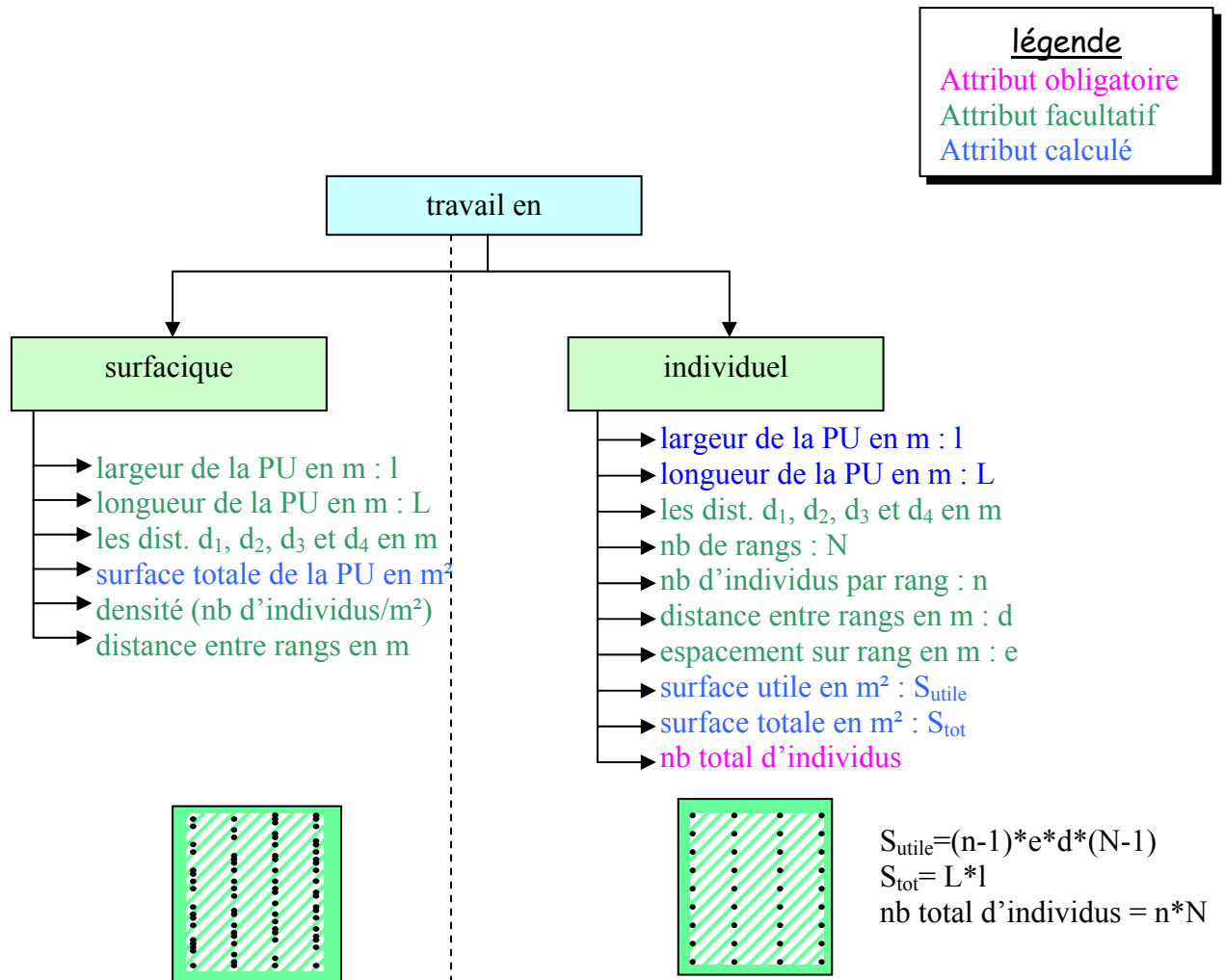
Figure 10 : Les attributs des PUs en mode surfacique et individuel
