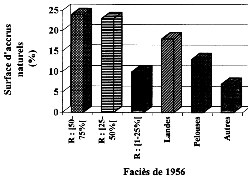
Figure 3 : Répartition des surfaces qui sont devenues des bois entre 1956 et 1991 en fonction du faciès de 1956 (R = Recouvrement arboré).
