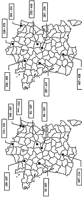
Cumul des températures - débournement du chêne en 1997 (début - fin) Stations météorologiques de référence
