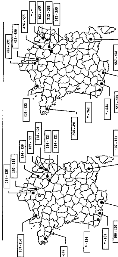
Cumul des températures - débournement du hêtre en 1997 (début - fin) Stations météorologiques de référence
