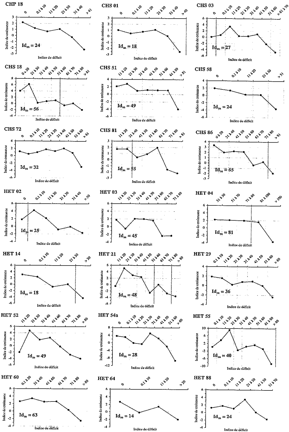
Figure 35. Evolution de l'indice de croissance radiale moyen par classe d'indice de déficit de réserve en eau pour les 9 peuplements de chênes et les 12 peuplements de hêtre présentant une corrélation significative entre la croissance et l'intensité du déficit. Pour chaque classe et chaque peuplement, les moyennes ont été calculées sur au moins trois années. Id_m correspond à l'indice de déficit hydrique moyen calculé sur toute la période (voir Tableau 20).
