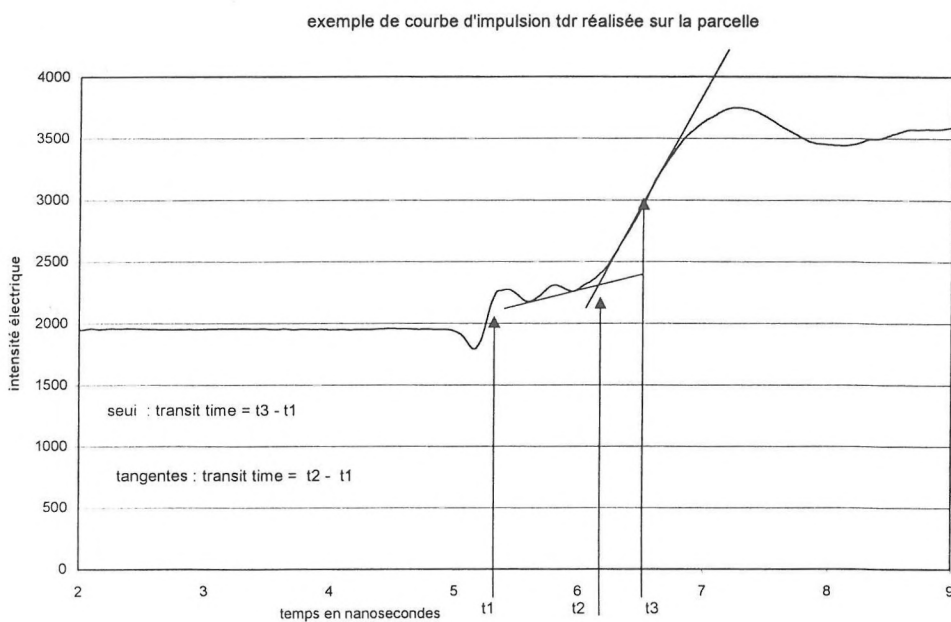
Figure 4 : Détermination de la fin du guide d'onde du TRIME
