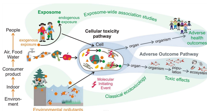
Figure. Les différentes voies des expositions chimiques des populations et des écosystèmes : conséquences (éco)-toxicologiques (voir rapport GT Toxicologie-Eco toxicologie, d'après Escher et al., 2017)
