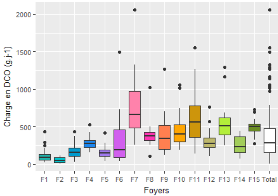
Figure 39 : Comparaison des charges journalières en DCO ( g.j^{-1} ) par ménage
