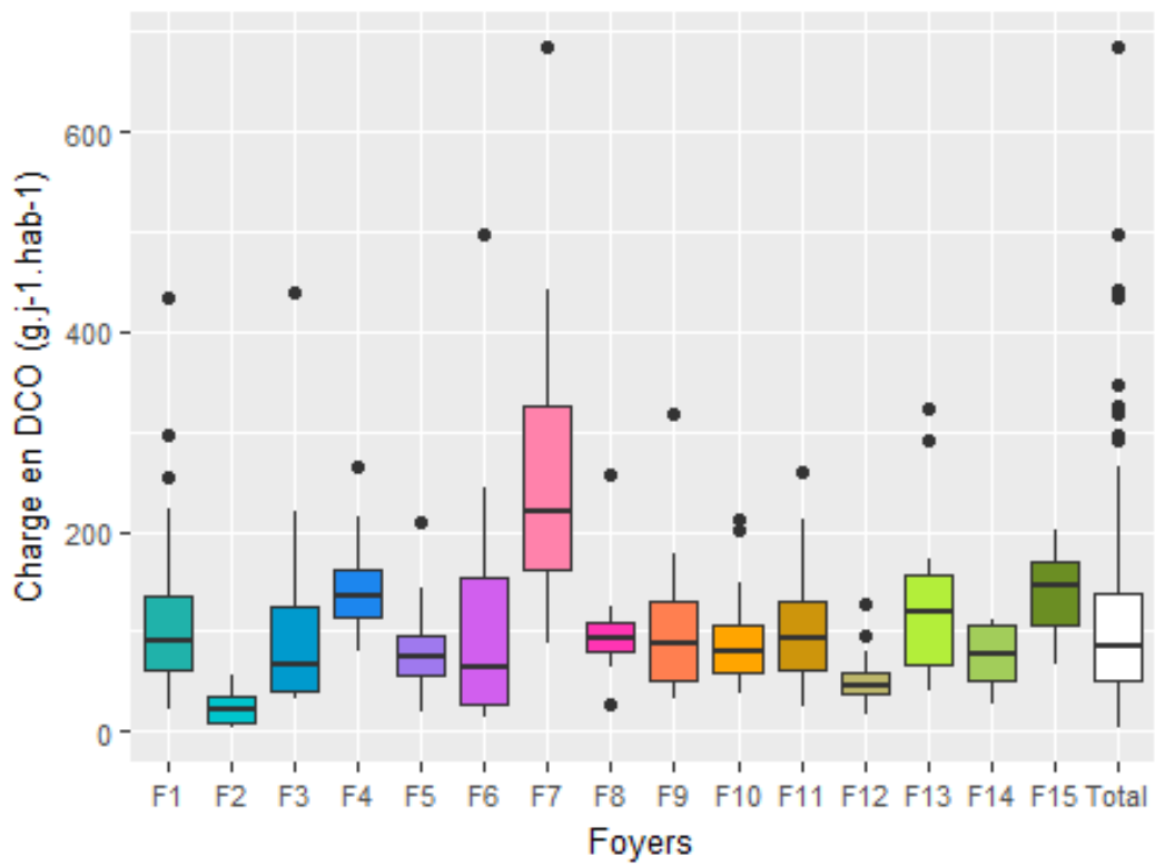
Figure 49 : Comparaison des charges journalières par habitant en DCO ( g.j^{-1}.hab^{-1} )
