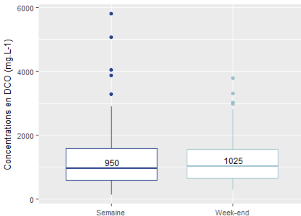
Figure 55 : Comparaison entre les concentrations en DCO (mg.L -1 ) des eaux usées d'un ménage pendant la semaine et le week-end
