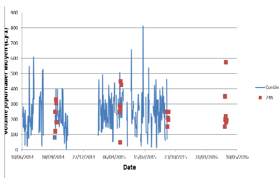
Figure 24 : Comparaison des volumes journaliers au sein du ménage F10
