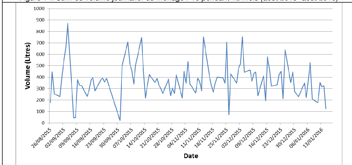
Figure 15: Suivi du volume journalier du ménage F17 pendant 12 mois (aout 2015- aout 2016)
