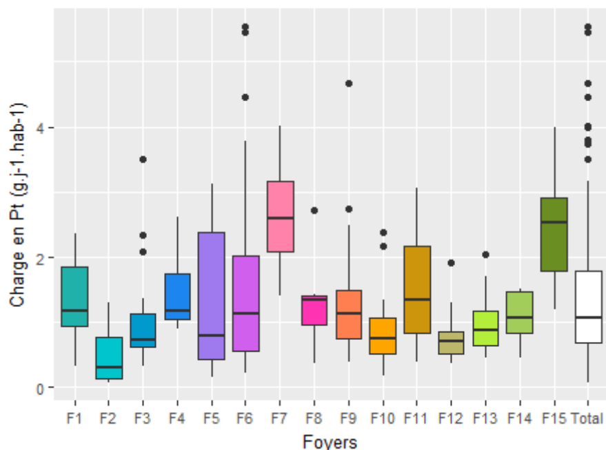
Figure 53 : Comparaison des charges journalières par habitant en Pt ( g.j^{-1}.hab^{-1} )
