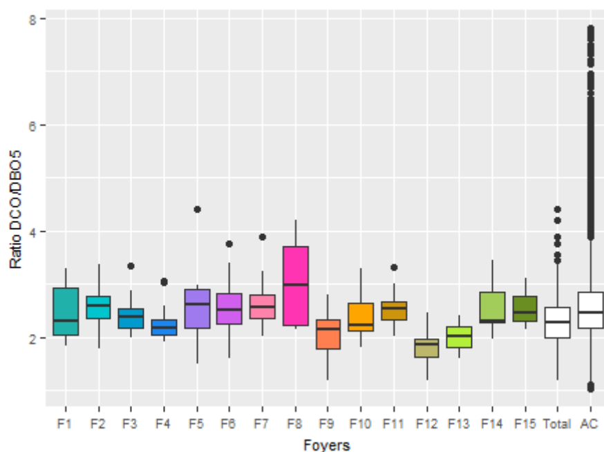
Figure 37 : Ratio DCO/DBO 5 des 15 ménages suivis, du jeu de données complet et des données de l'assainissement collectif
