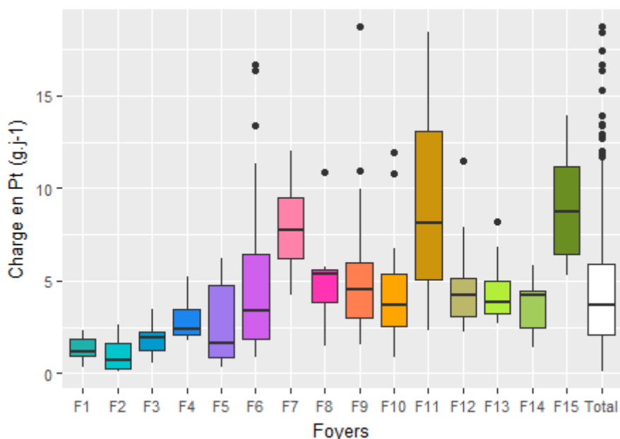
Figure 43 : Comparaison des charges journalières en Pt ( g.j^{-1} ) par ménage
