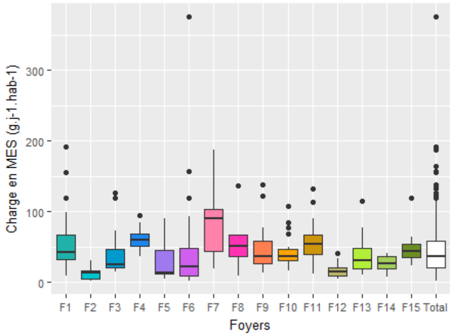
Figure 48 : Comparaison des charges journalières par habitant en MES ( g.j^{-1}.hab^{-1} )
