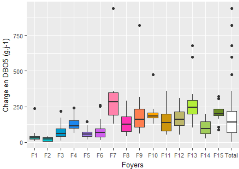
Figure 40 : Comparaison des charges journalières en DBO 5 ( g.j^{-1} ) par ménage
