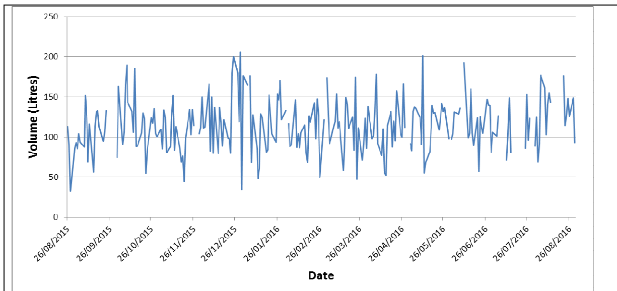
Figure 14: Suivi du volume journalier du ménage F16 pendant 12 mois (aout 2015- aout 2016)
