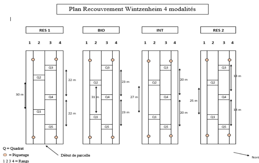
Figure 13 - Répartition des quadrats sur les parcelles de Wintzenheim (répétition n°2) (BUCHMANN, 2016)
