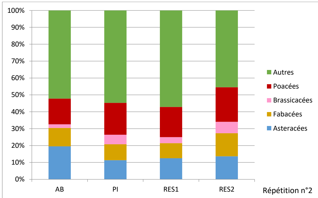
Figure 29 - Répartition des familles botaniques de 2016 à 2018 en fonction du recouvrement à Wintzenheim
