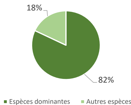
Figure 28 - Pourcentage du recouvrement espèces de 2016 à 2018 sur la base de 3 relevés (sans prendre en compte le sol nu)
