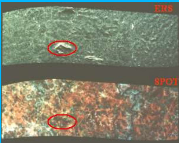
Figure 2 : Exemple illustrant la détectabilité par ERS et non par SPOT des régoïthes sur le bassin de Siguiri (frontière Mali/Guinée).
