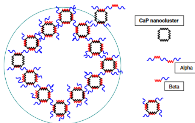
Figure 5: modèle de croissance des micelles de caséines.
