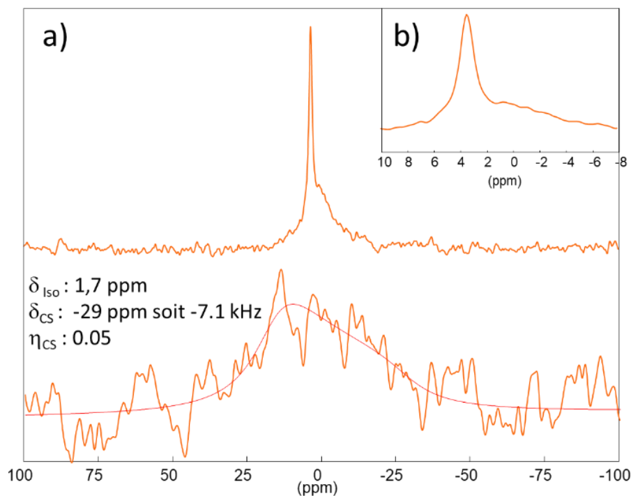
Figure 19:a) Spectres ZG et CP obtenus sur le PPCN 60 g/L+TG et déminéralisé puis additionné de CaCl_2 , b) zoom du spectre ZG.
