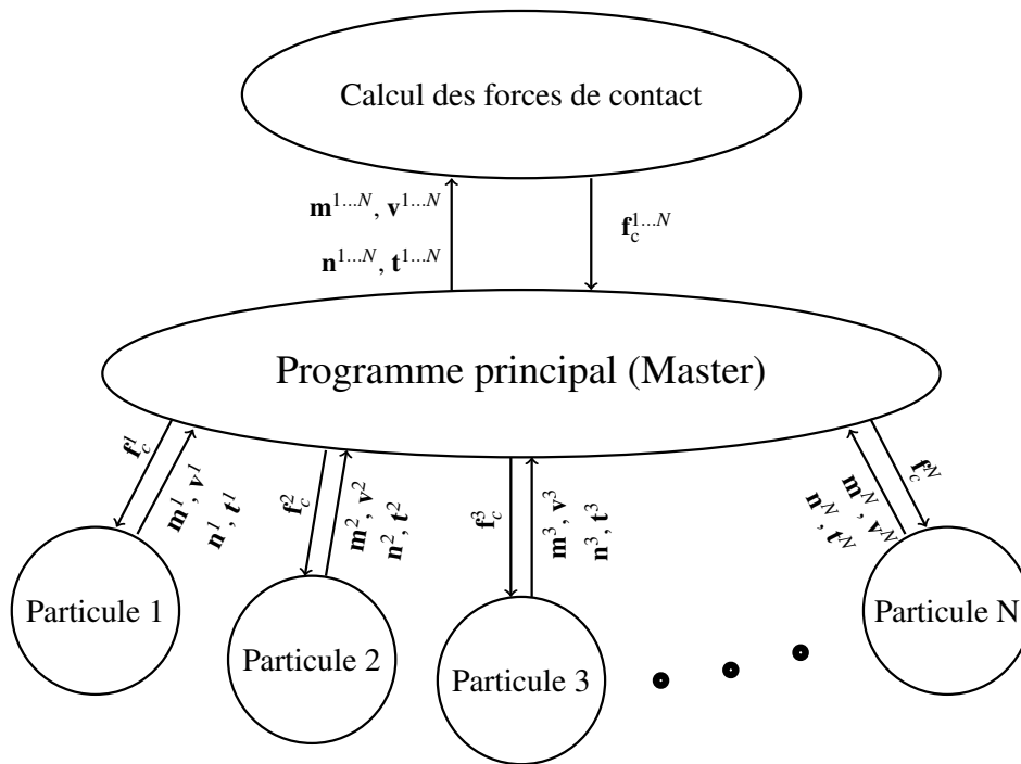
FIGURE 1 – Schéma de la procédure de parallélisation de l'approche MPM-CD ; N est le nombre de particules, et f_c , m , n et t représentent, respectivement, les vecteurs de force de contact, de masse, normal et tangentiel, pour le noeud de contact potentiel de chaque particule.
