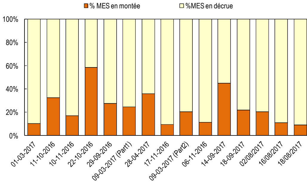
Figure 23 – Répartition de la quantité de MES transportée entre la montée de crue et la décrue - rivière Pérou
