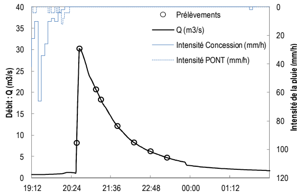
PONT rivière Pérou : crue du 06/11/2016 – type C
