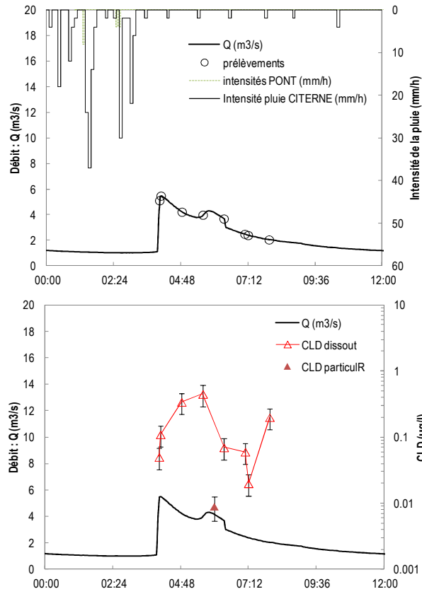
PONT rivière Pérou : Crue du 01/03/2017 – type A
