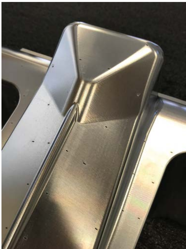
DÉTAIL DU BUSAGE SUR UN OUTIL DE THERMOFORMAGE PAR STRATOCONCEPTION.
