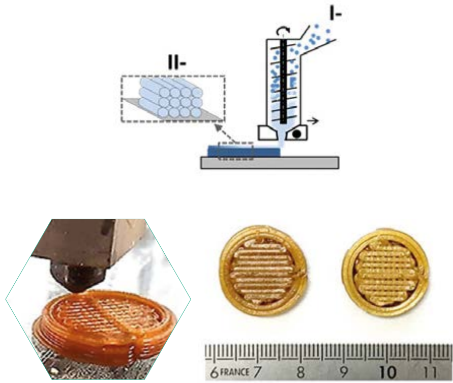
Figure 4. Schéma d'illustration de l'imprimante 3D FA-DFF par extrusion-dépôt et impression 3D de la zéine plastifiée : extrusion (I-) simultanée au dépôt de fondu (II-) (a-). Zéine à l'état fondu en sortie de filière ( \varnothing_{\text{filière}} = 1\text{ mm} ; V_{\text{dépôt}} = 2\text{ mm}\cdot\text{s}^{-1} ) et obtention de pièces imprimées cohésives, telles que des pastilles pharmaceutiques modèles, par l'adhésion des filaments juxtaposés et superposés ( \varnothing_{\text{pastille\_modèle}} = 20\text{ mm} , h_{\text{pastille\_modèle}} = 4,8\text{ mm} -soit 8 couches de filament superposées, avec un pas de déplacement vertical de 0,6 mm- ; b- et c-). Collaboration : INRAE Pays de Loire, BIA/GEPEA/CompositIC-IRD.
