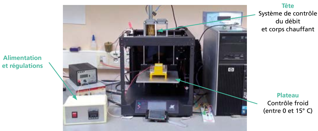
Figure 6. Imprimante 3D commerciale modifiée pour l'impression d'aliments fonctionnels.
